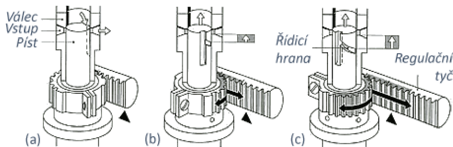
Obr. 10 - Natáčení pístu regulační tyčí: (a) - nulová dodávka, (b) - částečná dodávka, (c) - maximální dodávka. [8]
