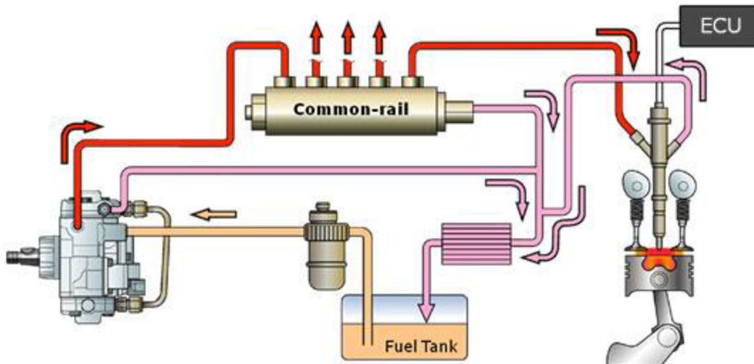
Obr. 2 - Schéma vstřikování Common rail s vysokotlakou i nízkotlakou regulací [5]
