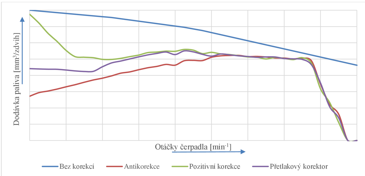
Obr. 11 – Průběh dodávky paliva v závislosti na činnosti korektorů
