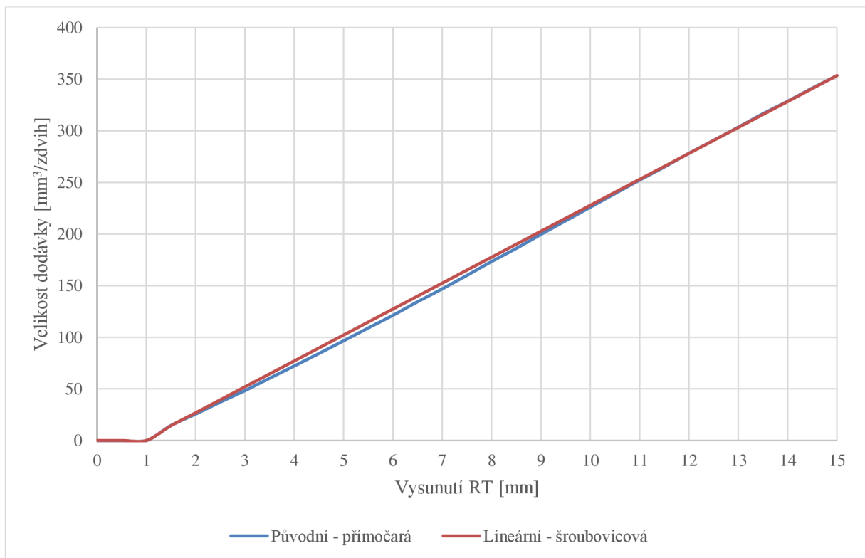
Obr. 65 - Graf závislosti velikosti dodávky paliva na vysunutí regulační tyče
