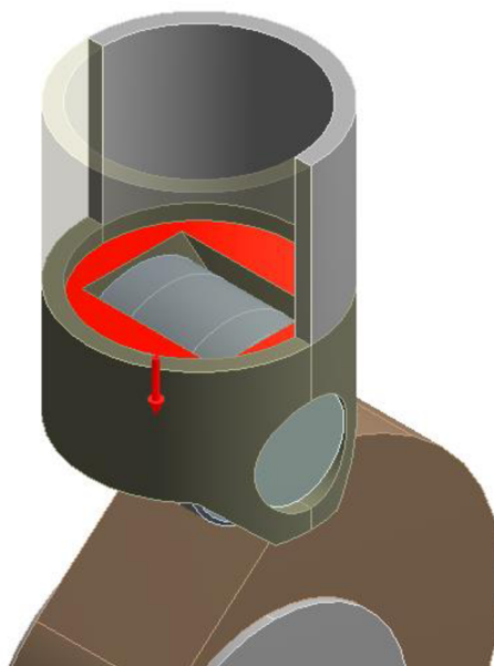
Obr. 54 - Zatížení zvedáku
