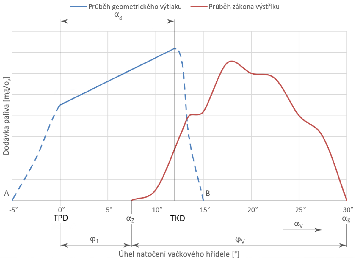
Obr. 1 - Průběh geometrického výtlaku a příslušného zákona vstřiku [2]
