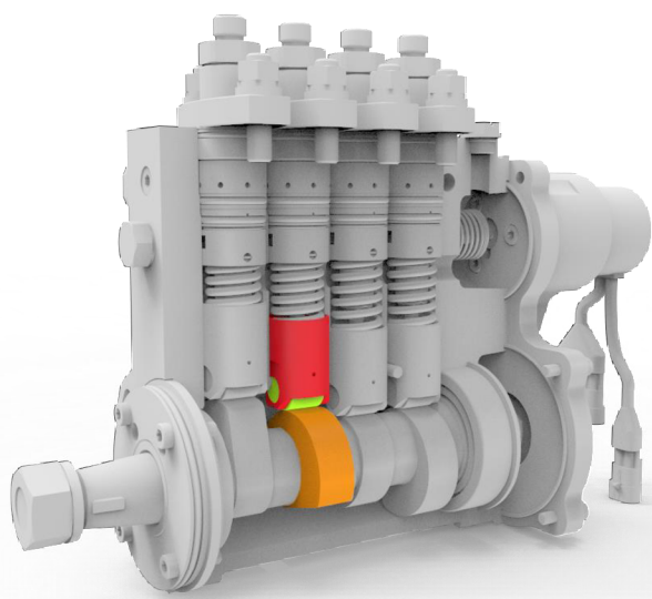
Obr. 30 – Model čerpadla Mj
