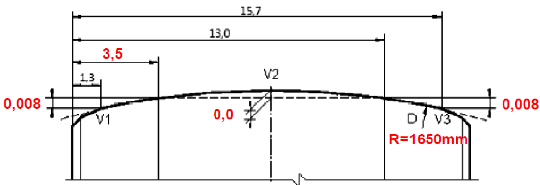
Obr. 34 - Profil kladky dle naměřených hodnot - zvýrazněné kóty byly upraveny dle výsledků měření.
