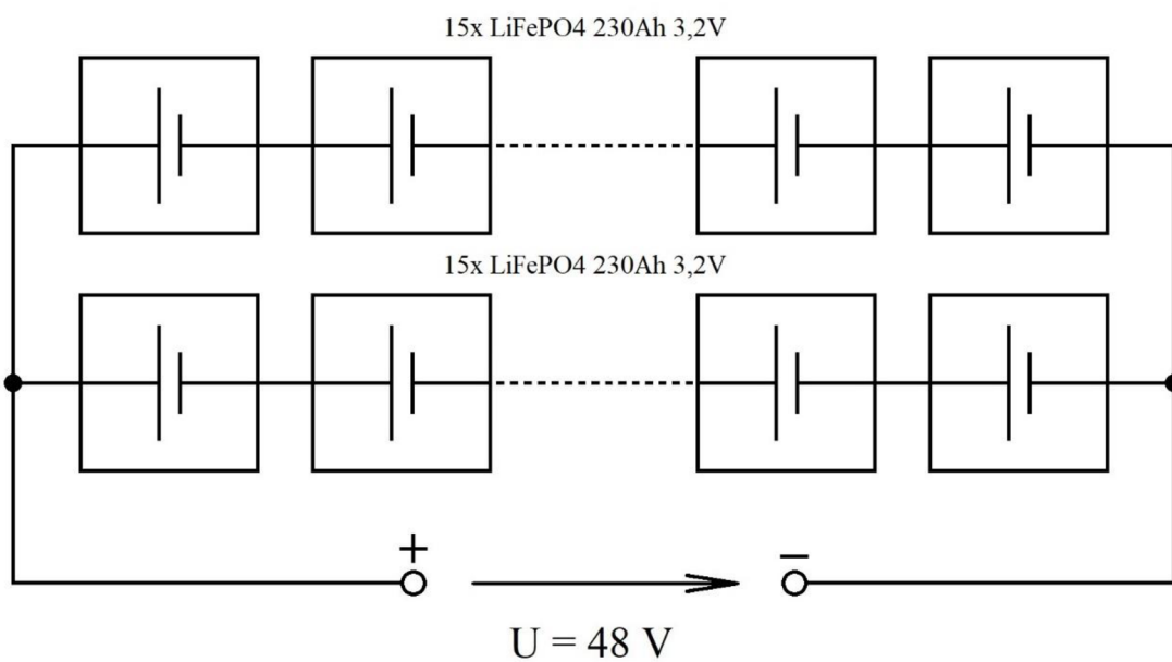
Obrázek 22 - Zapojení akumulátorů
