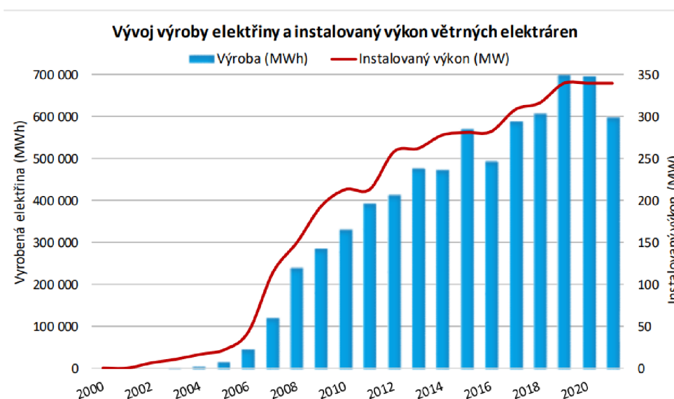
Graf 2 - Vývoj výroby elektrické energie a instalovaného výkonu VTE v ČR [8]
