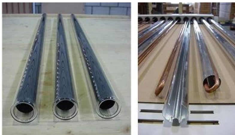
Obrázek 17: Trubkový dvojitý vakuový kolektor na bázi Sydney trubek s teplosměnnou lamelou [11]
