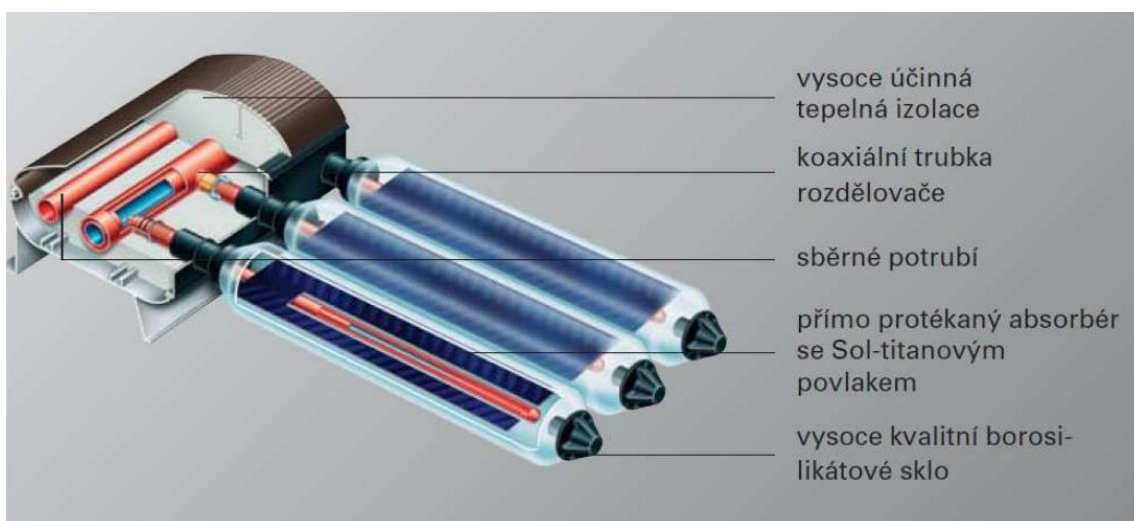
Obrázek 15: Vakuové trubice s přímo protékajícím absorberem [13]
