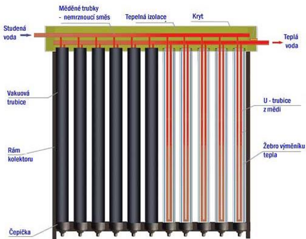
Obrázek 18: Schéma trubkového dvojitýho (Sydney) vakuového kolektoru
