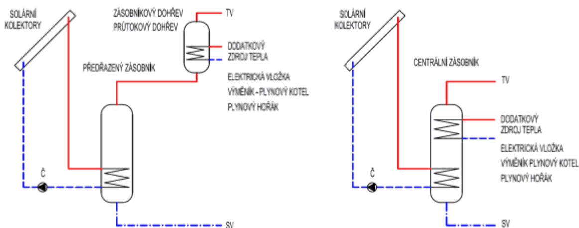
Obrázek 5: Schéma solární přípravy teplé vody pro rodinný dům: vlevo – s předehřivacím zásobníkem, vpravo – s bivalentním zásobníkem [4]
