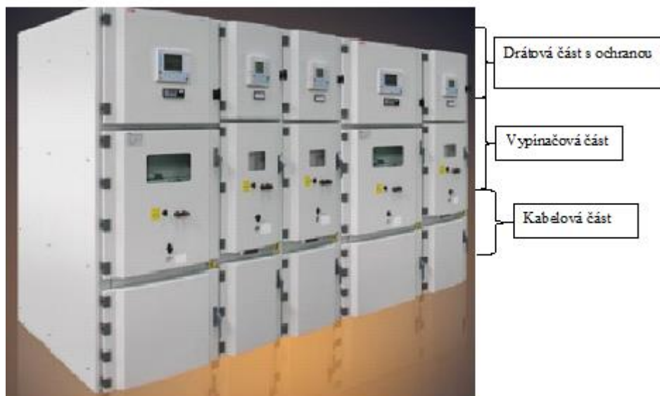
Obrázek 1. Příklad vzduchově izolované rozvodny vysokého napětí firmy ABB [1]
