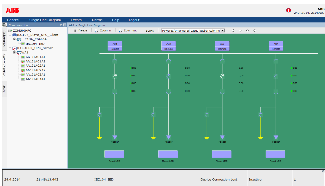
Obrázek 22. Správnost připojení demo panelu
