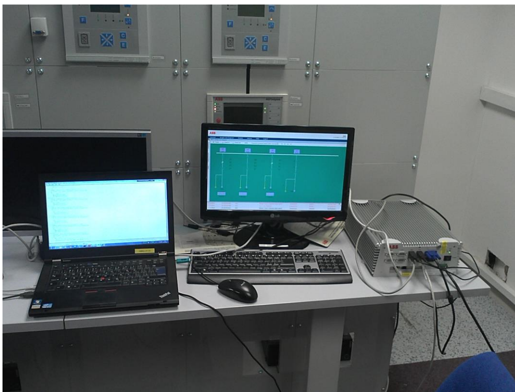
Obrázek 19. Testování konfigurací řídicího systému COM600
