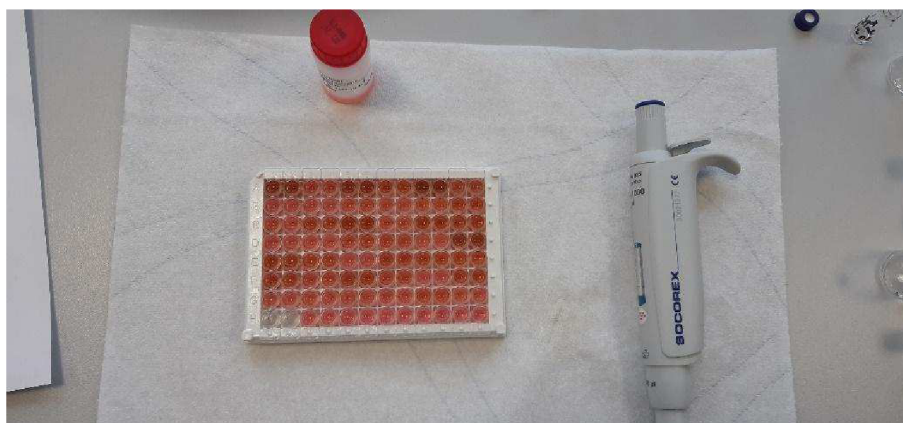
Obrázek č. 7: Po přidání konjugátu, růžový kolorit buněk Foto: Ing. Hana Süßenbeková
