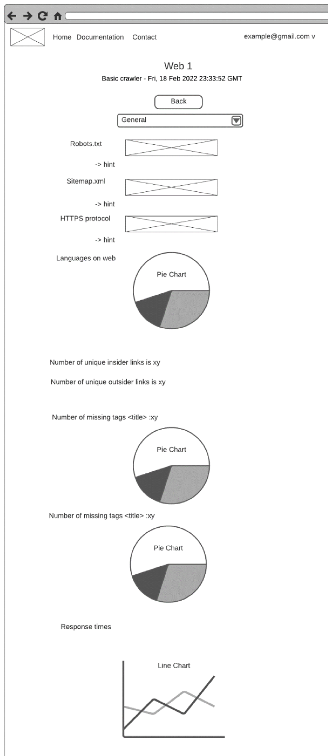
Obrázek 7: Basic crawler detail 1 – logický design
