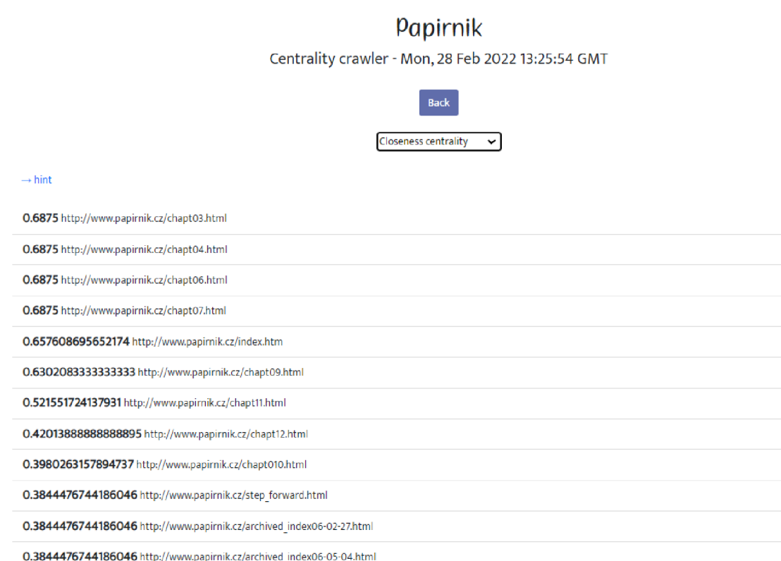
Obrázek 17: Ukázka výstupní obrazovky Centrality crawler 1
