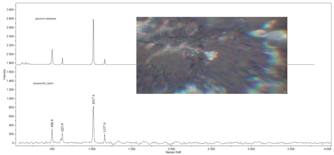
Obrázek 3.13 Ramanova spektra a EM zobrazení \text{CaSO}_4 ve vzorku M3.
