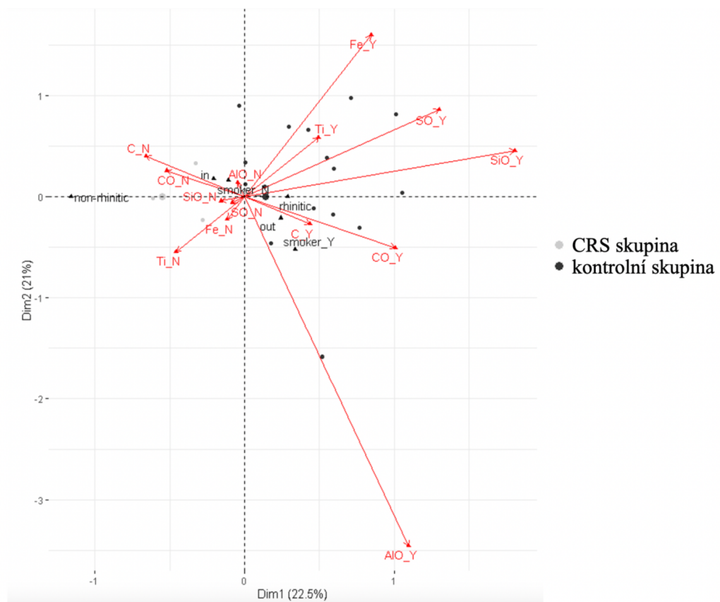
Obrázek 3.16 MCA biplot. Upraveno podle Čabanové a kol. (97).
