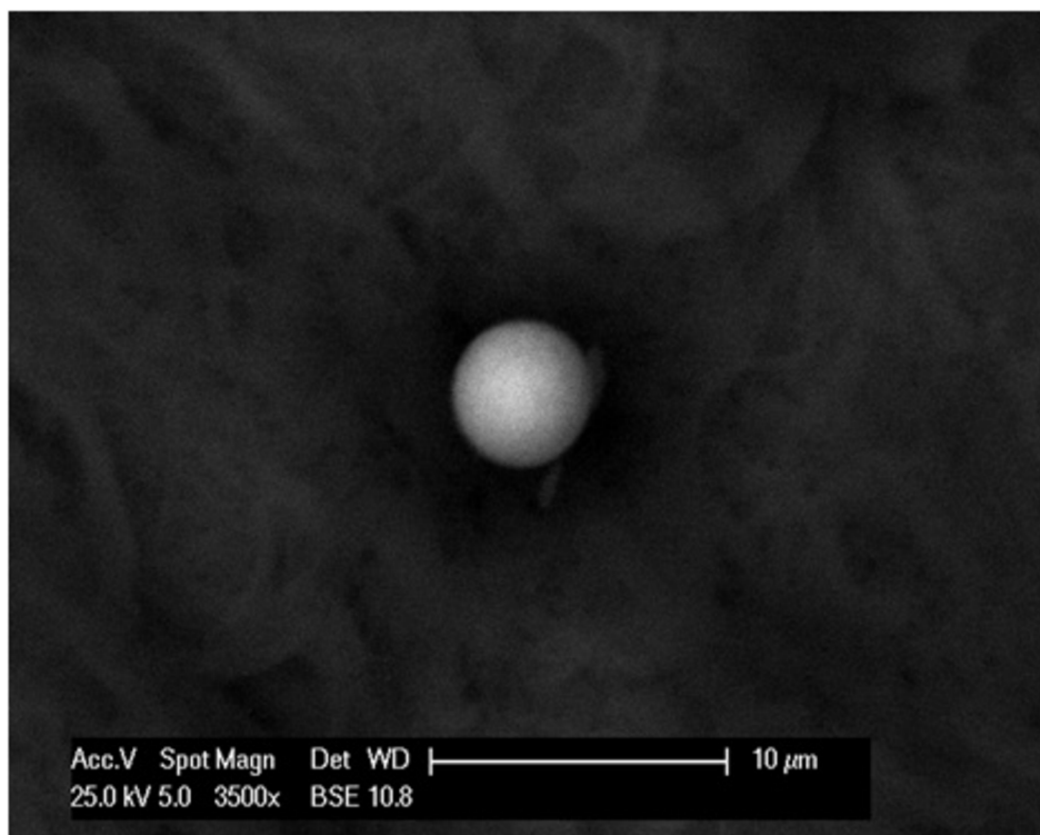
Obrázek 3.8 Kulovitá částice železa ve vzorku M1 v obrazu SEM (zvětšení 3500x).
