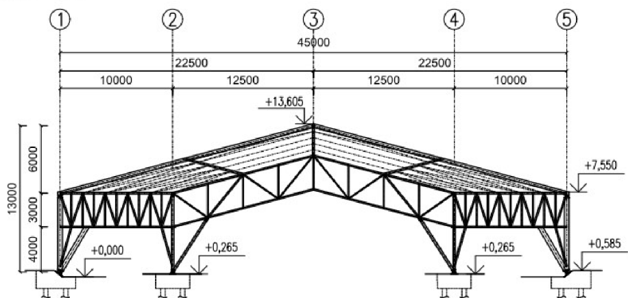
POHLED VÝCHODNÍ/ZÁPADNÍ
