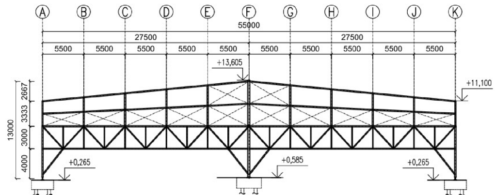
POHLED VÝCHODNÍ/ZÁPADNÍ
