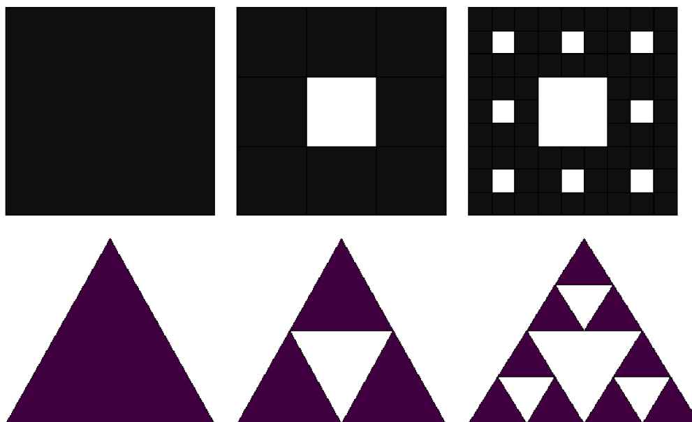
Obrázek 3.8: Ukázka prvních dvou iterací Sierpinského koberečku a Sierpinského trojúhelníku.
