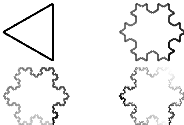
Obrázek 3.10: Ukázka tří iterací Kochovy vložky.
