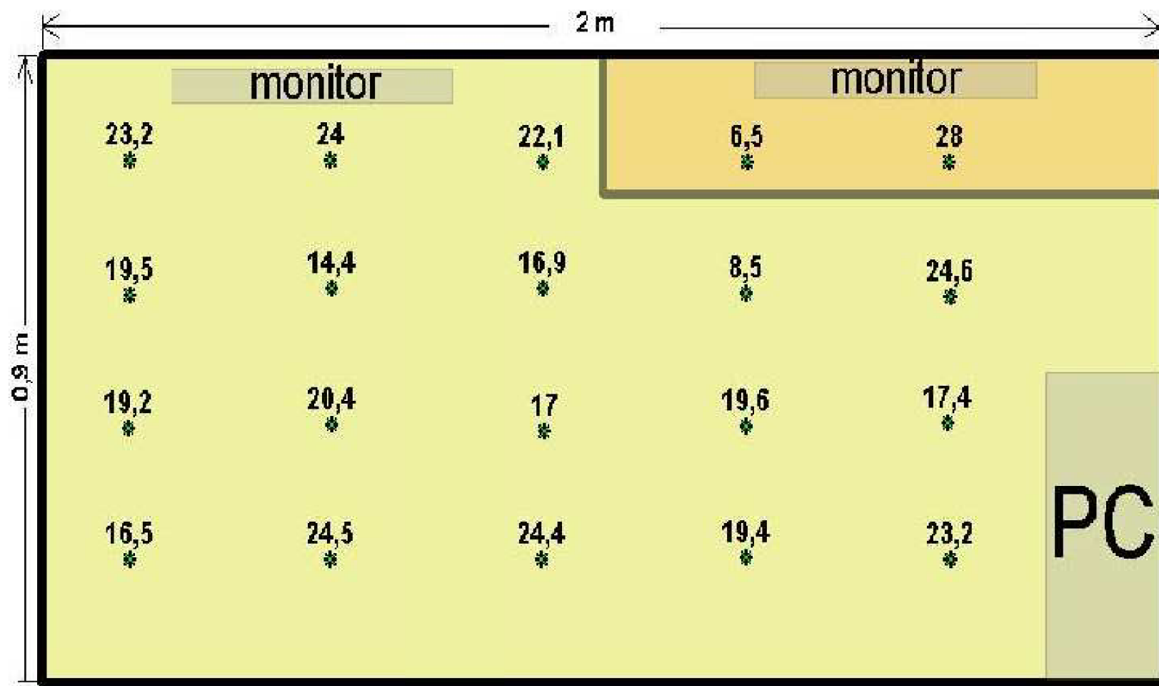
Obrázek 22: Rozložení měřících bodů na pracovním stole s počítačem
