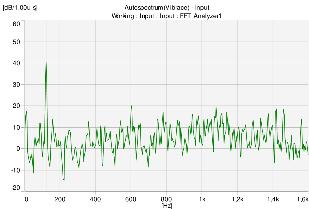
Obrázek 15: Spektrum vibrací při měření krytu PC
