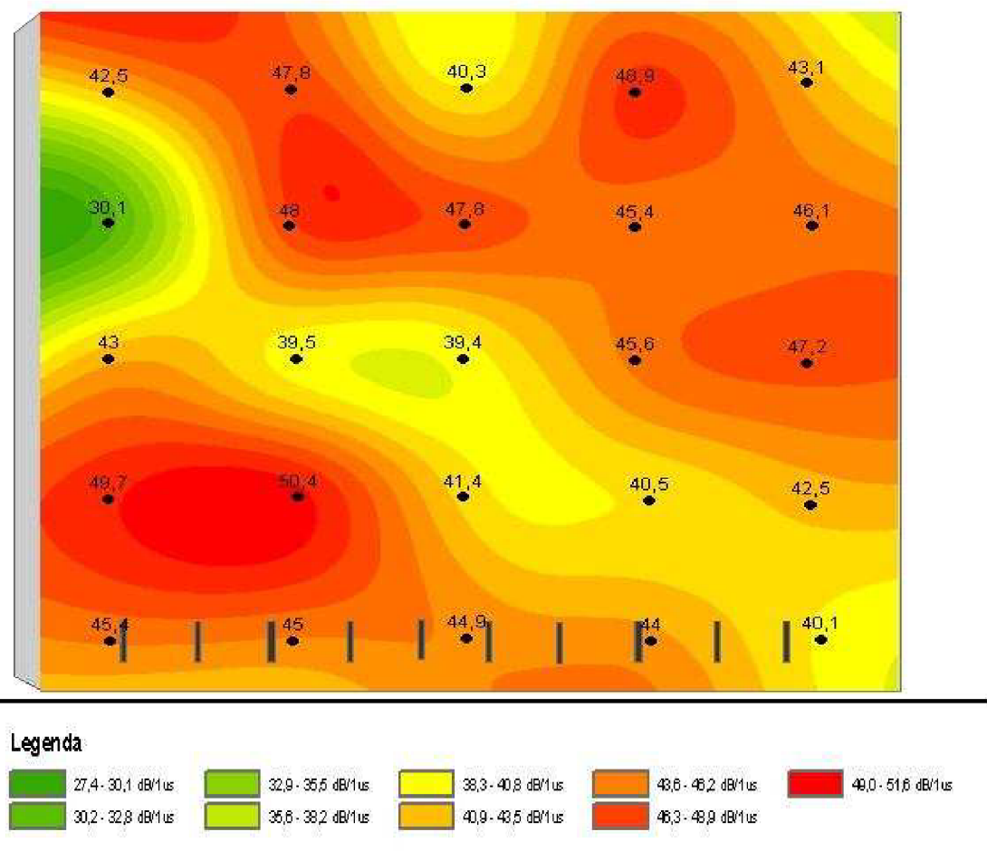
Obrázek 19: Vibrační mapa pravého boku kryt počítače
