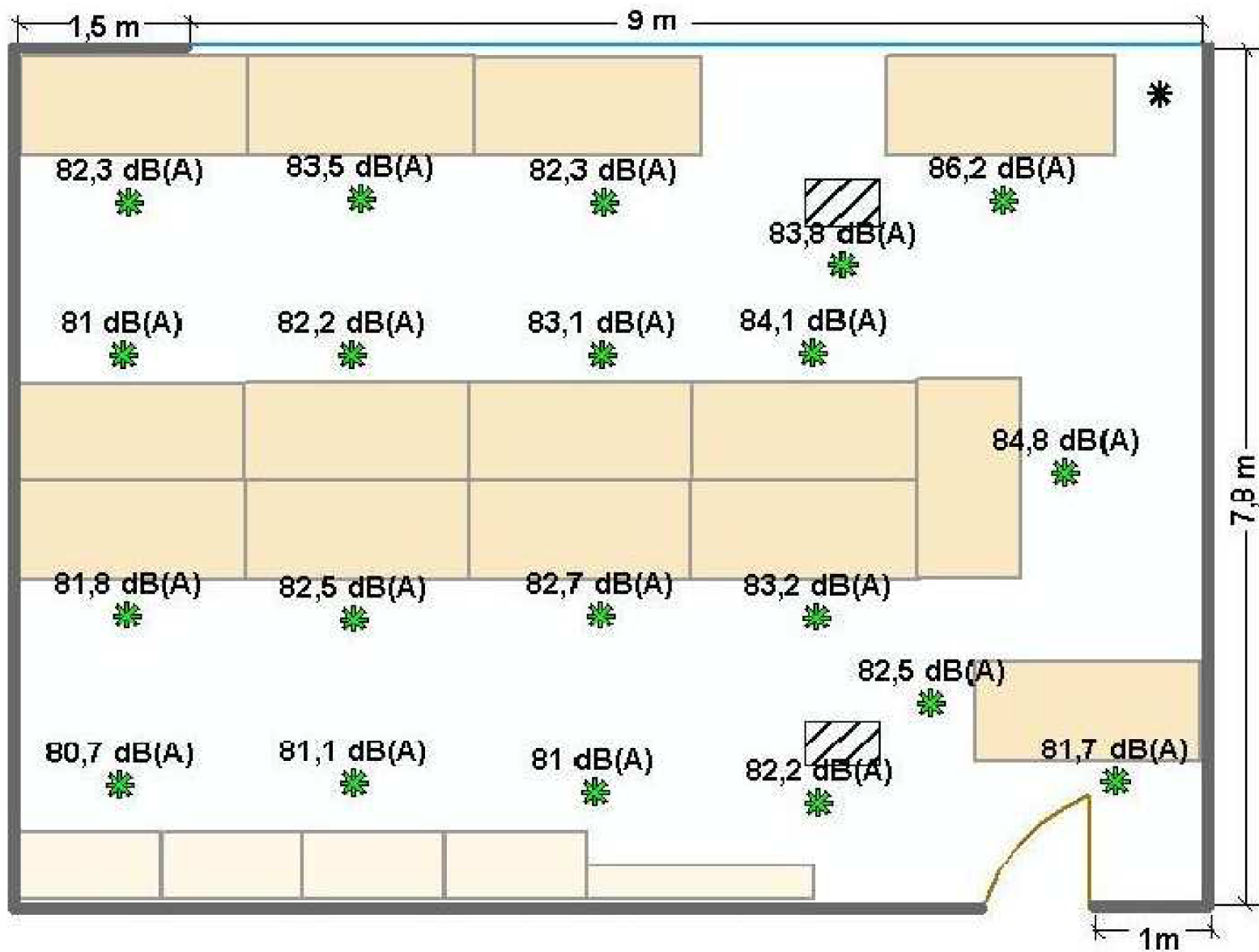
Obrázek 11: Rozložení měřících bodů pro místnost E237
