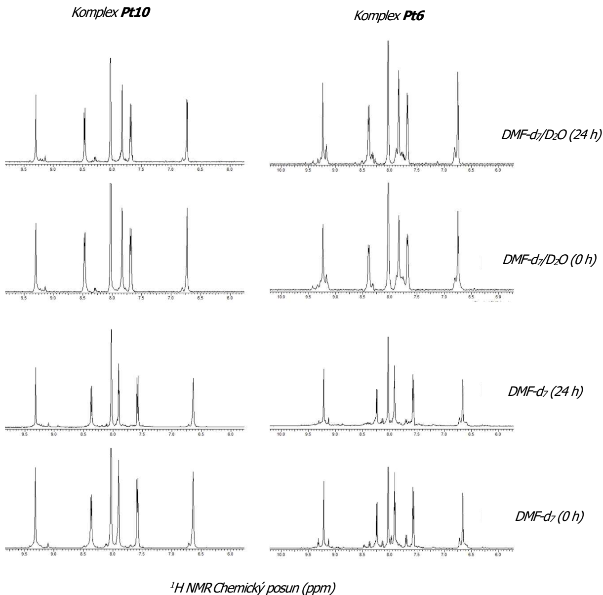
Obr. č. 38: 1 H NMR měření stability a hydrolytické stability reprezentativních komplexů Pt10 a Pt6
