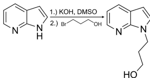
Obr. 29: Schéma N1 -modifikace 7-azaindolu navázáním propanolu (derivát O1 )
