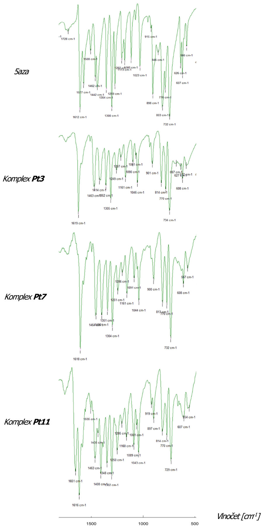
Obr. 36: Porovnání FTIR spekter 5aza a jeho komplexů Pt3, Pt7 a Pt11.
