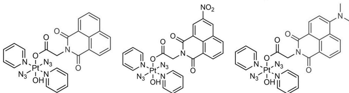
Obr. 22: Strukturí vzorce monofunkcionalizovaných fotoaktivovatelných komplexů (zleva) trans,trans,trans -[Pt(py) 2 (N 3 ) 2 (OH)(gly-3-H-Nap)], trans,trans,trans -[Pt(py) 2 (N 3 ) 2 (OH)(gly-3-NO 2 -Nap)] a trans,trans,trans -[Pt(py) 2 (N 3 ) 2 (OH)(gly-4-NMe 2 -Nap)] (převzato z [132]; upraveno)
