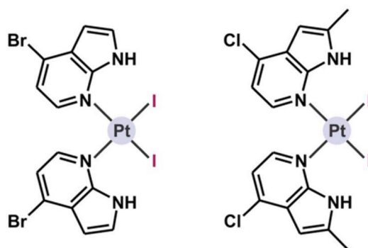
Obr. 14: Strukturální vzorce cis-[Pt(4Br-7aza) 2 I 2 ] a cis-[Pt(2Me4Cl-7aza) 2 I 2 ] (převzato z [89])
