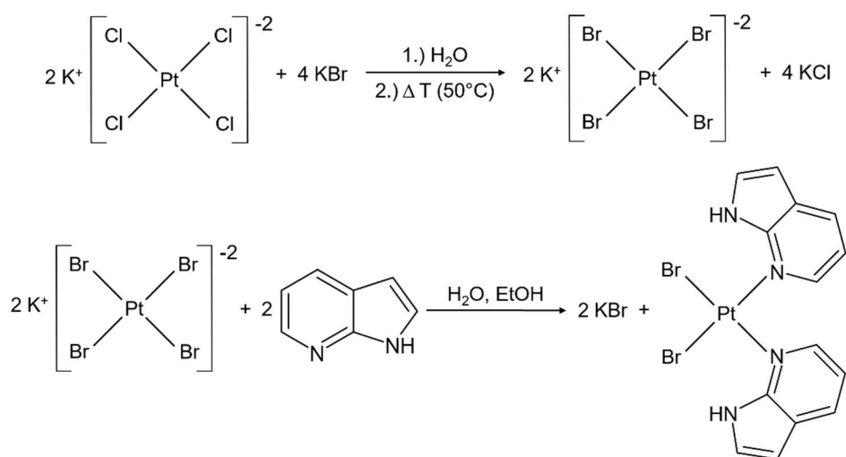
Obr. 25: Reakční schéma syntézy komplexu cis -[Pt(7aza) 2 Br 2 ] ( Pt5 )
