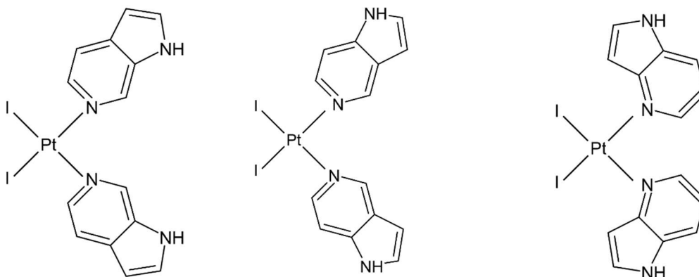
Obr. 28: Strukturní vzorce komplexů (zleva) cis -[Pt(6aza) 2 I 2 ] ( Pt10 ), cis -[Pt(5aza) 2 I 2 ] ( Pt11 ) a cis -[Pt(4aza) 2 I 2 ] ( Pt12 ).
