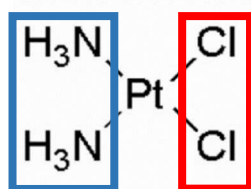
Obr. 1: Strukturní vzorec cisplatinu s vyznačením typu ligandů – modré (carrier, neodstupující ligandy), červené (odstupující ligandy) (převzato z [20]; upraveno)
