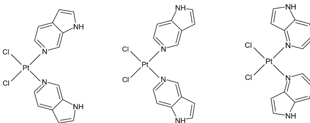
Obr. 24: Strukturní vzorce komplexů (zleva) cis -[Pt(6aza) 2 Cl 2 ] ( Pt2 ), cis -[Pt(5aza) 2 Cl 2 ] ( Pt3 ) a cis -[Pt(4aza) 2 Cl 2 ] ( Pt4 ).
