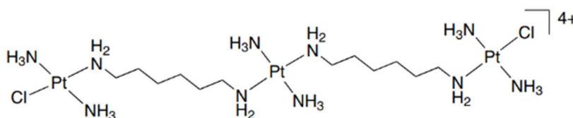
Obr. 6: Trinukleární komplex BBR3464 [ \{trans-PtCl(NH_3)_2\}_2-\mu-trans-Pt(NH_3)_2\{NH_2(CH_2)_6NH_2\}_2\}^{4+} (převzato z [62])
