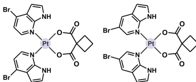
Obr. 18: Strukturální vzorec [Pt(4Br-7aza)_2(cbdc)] a [Pt(5Br-7aza)_2(cbdc)] (převzato z [89])
