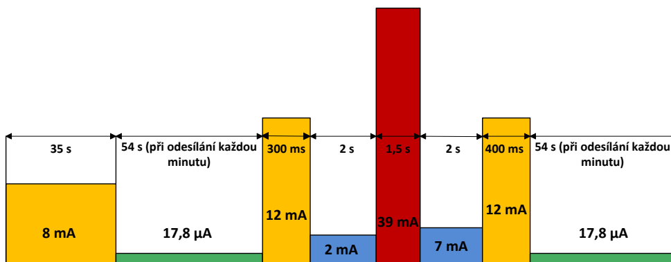
Obr. 6.3: Graf spotřeby Indoor senzoru.
