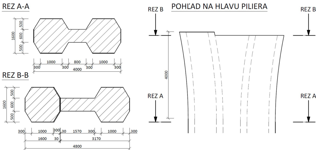
Obrázok 4. 1: Prierez piliera
