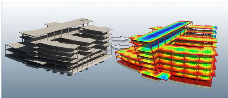
Obrázek č. 8 Ukázka statické pevnostní analýzy
