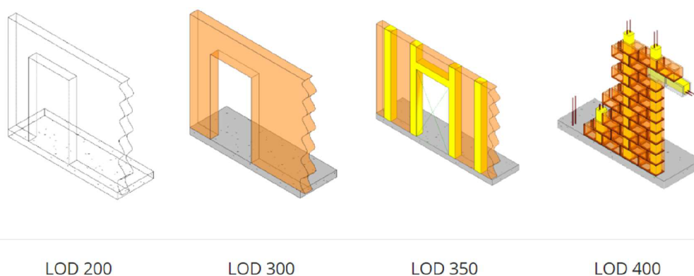
Obrázek č. 13 Grafické podoby LOD pro stěnu [BIMforum]
