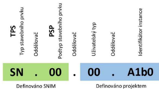
Obrázek č. 23 Struktura kódu SNIM [40]
