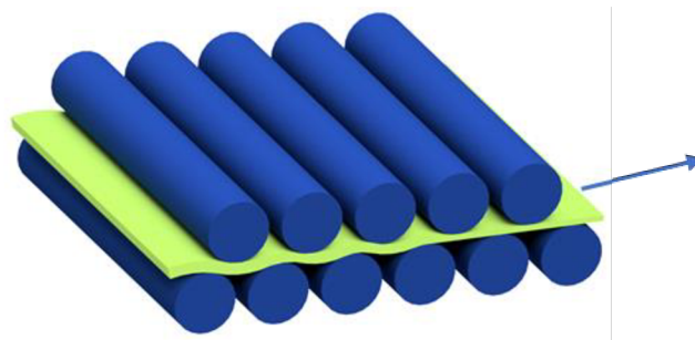
Obr. 2.24 Rovnění mezi válci
