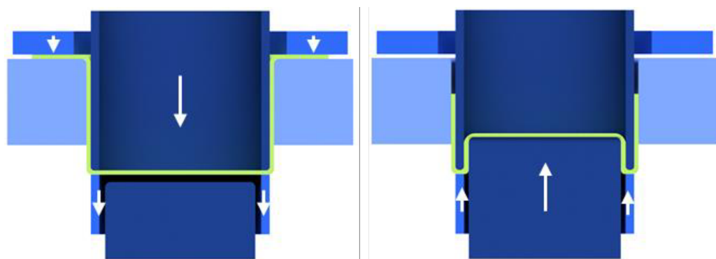
Obr. 2.28 Zpětné tažení
