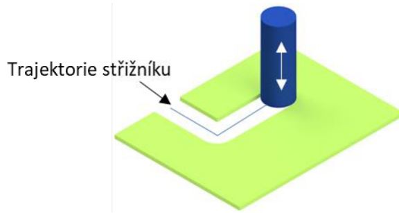
Obr. 2.13 Prosekávání
