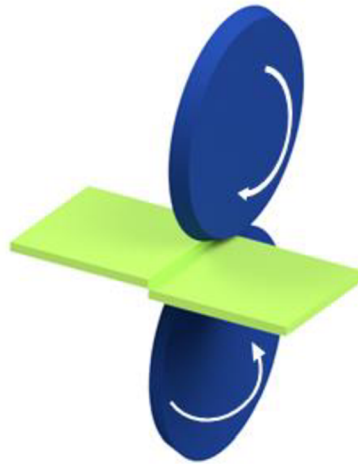
Obr. 2.10 Prosté stříhání dvěma kotoučovými břity
