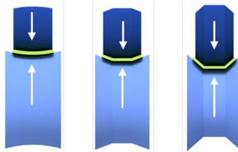
Obr. 2.23 Kontinuální ohýbání
