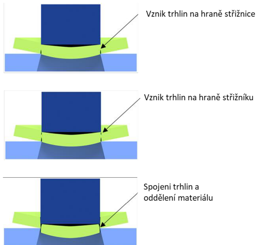
Obr. 2.1 Fáze stříhu
