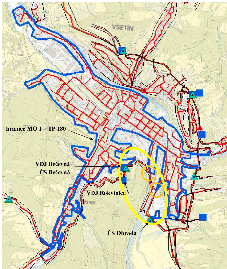
Obr. 44 Měřicí okrsek č.1 – napájecí uzel VDJ Bečevná, TP 180
