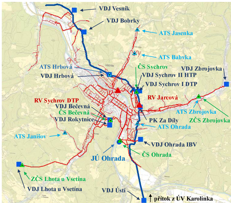
Obr. 23 Přehledné schéma vodovodní sítě Vsetín
