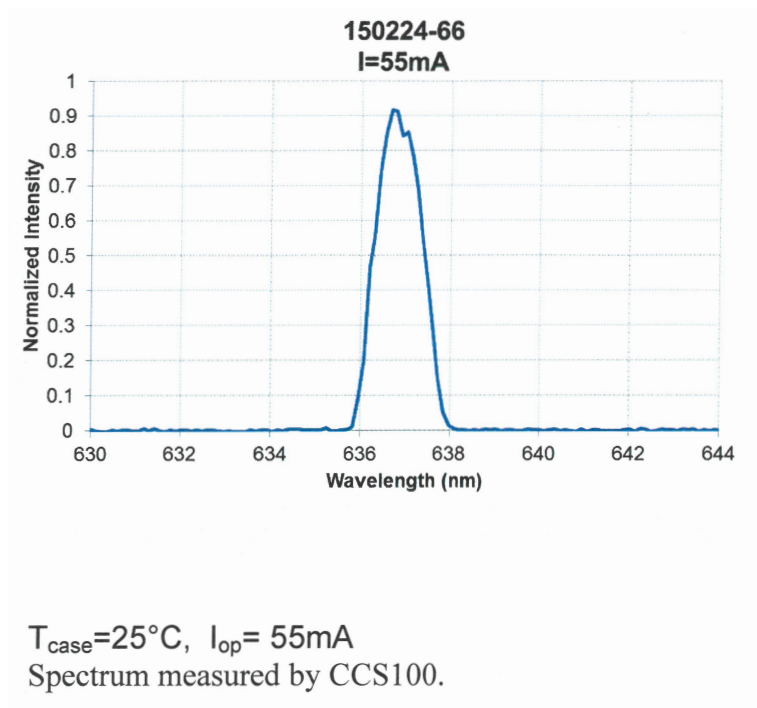
Obr. 5.1: Spektrum laserové diody, které bylo udávané na datovém listu
