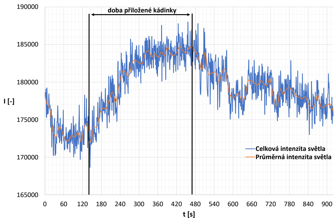
Obr. 6.7: Závislost intenzity světla na čase před a po přiložení kádinky s vodou 24 °C
