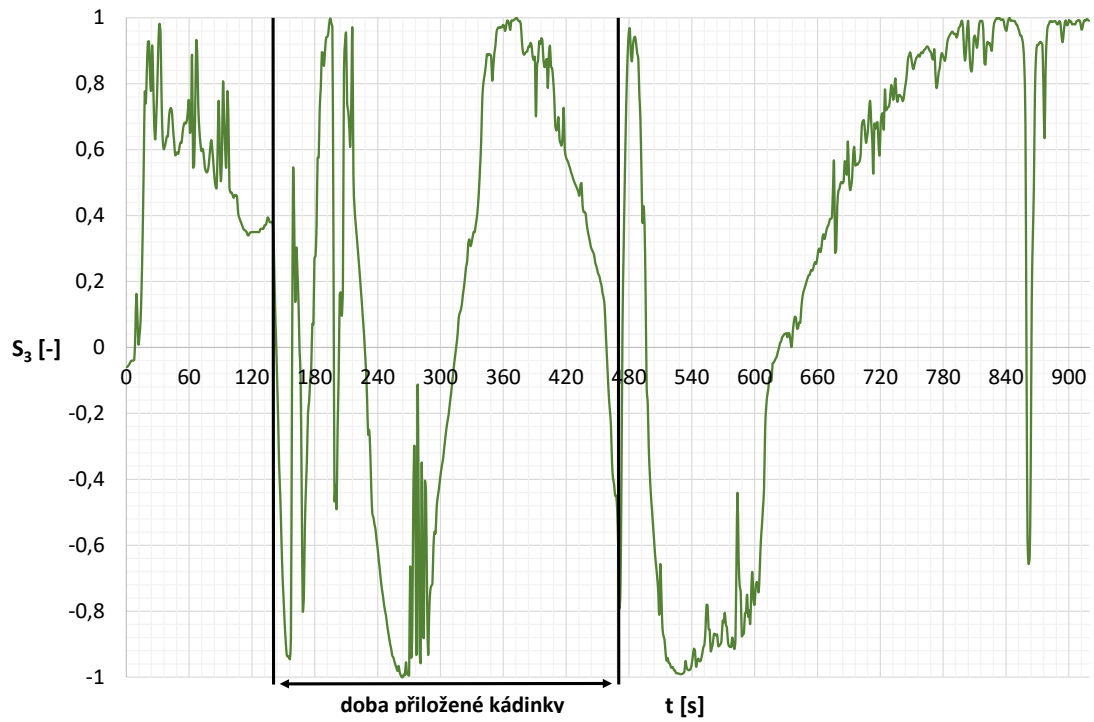
Obr. 8.3: Závislost Stokesova vektoru S_3 při teplotě 48\text{ }^\circ\text{C}
