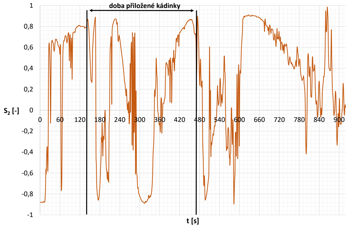
Obr. 8.2: Závislost Stokesova vektoru S_2 při teplotě 48 °C
