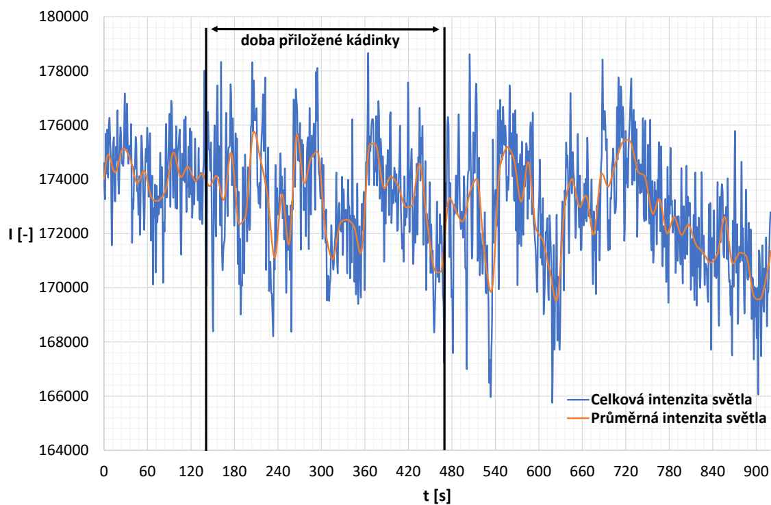
Obr. 7.9: Závislost celkové a průměrné intenzity světla na čase při teplotě 0 °C
