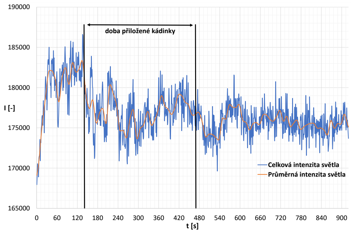
Obr. 8.9: Závislost celkové a průměrné intenzity světla na čase při teplotě 48 °C
