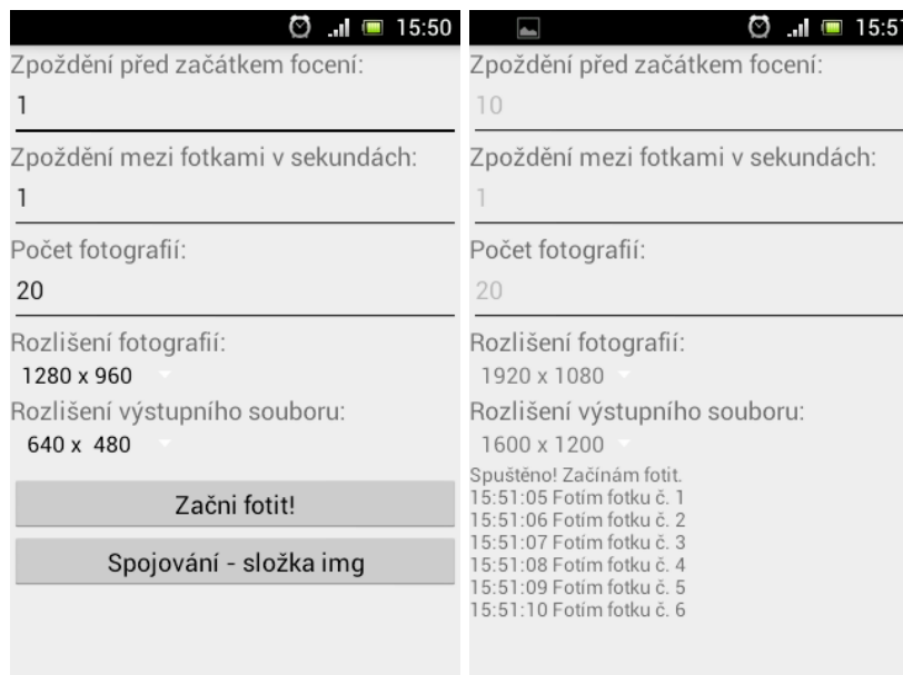
Obrázek 4.6: Ukázky uživatelského rozhraní aplikace – vlevo vzhled hned při startu, vpravo vzhled při pořizování fotografií. (vlastní práce)
