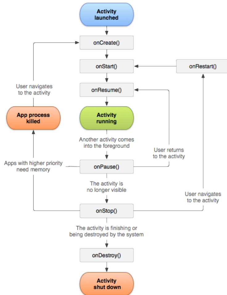
Obrázek 3.3: Schéma životního cyklu aktivity. Převzato z [10].
