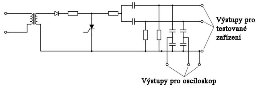
Obr. 5-3 Schématické znázornění rázového generátoru
