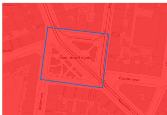
Obrázek 47: Četnosti výskytu bezvětří v Praze Zdroj: iprpraha.cz
