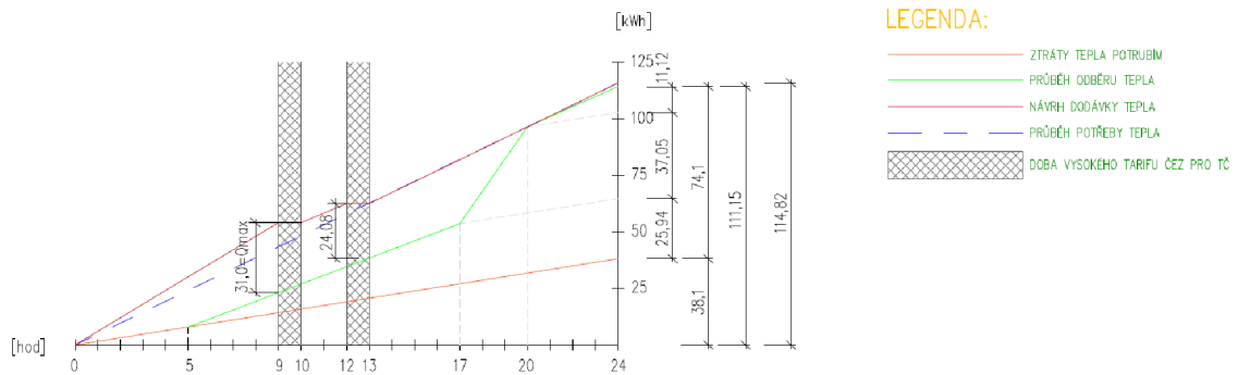
Obr. 30 Graf denní potřeby a dodávky tepla
