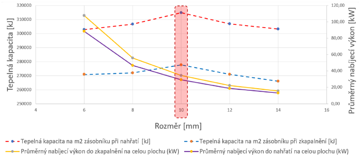
Obr. 14 Poměr tepelné kapacity k nabíjecím výkonům
