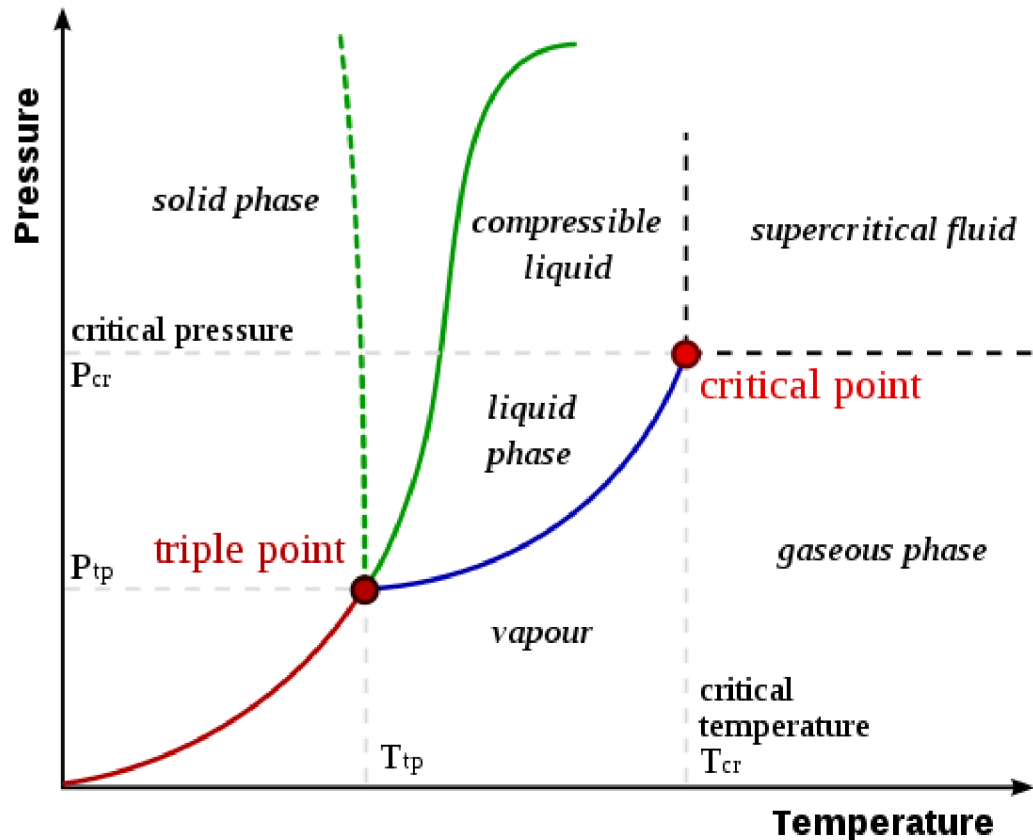
Obr. 4 Fázový diagram [10]
