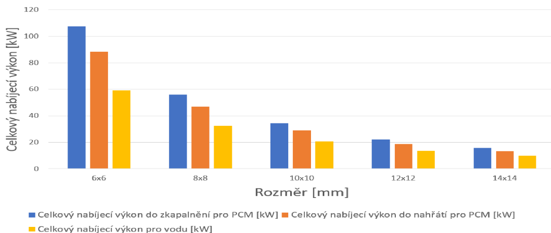
Obr. 16 Porovnání celkových nabíjecích výkon
