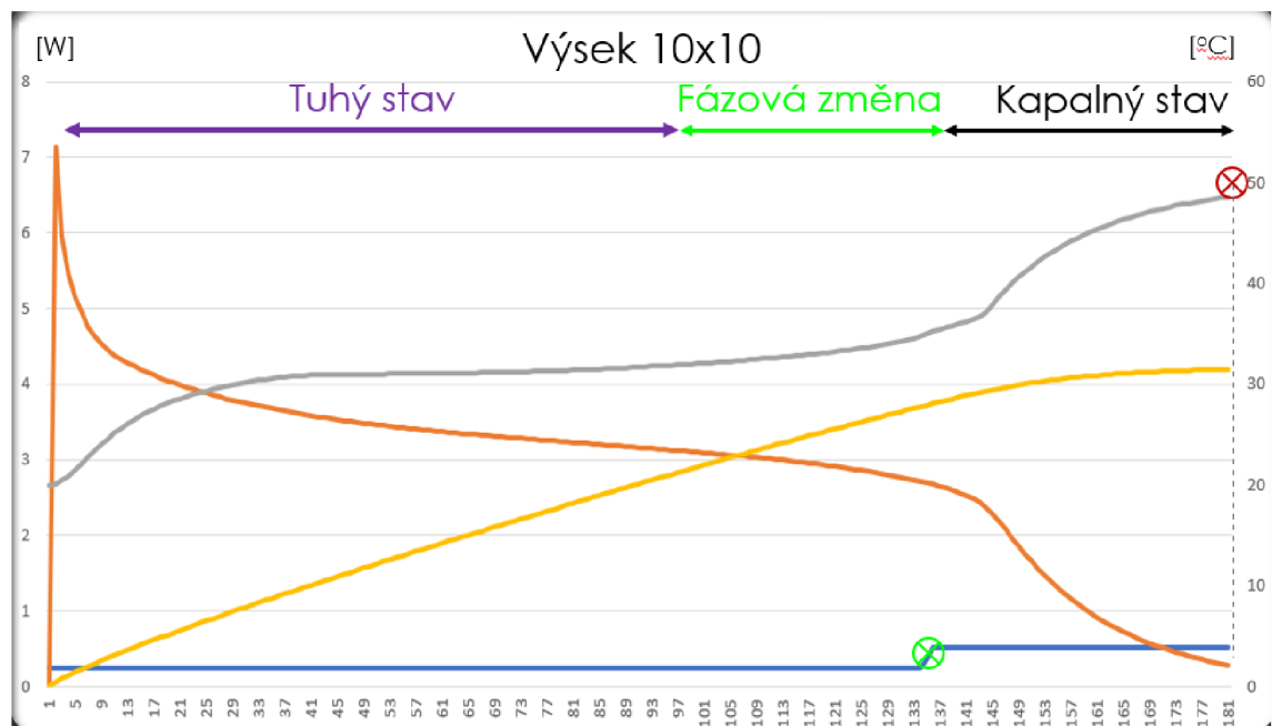
Obr. 13 Závislost vlastností PCM pro výsek 10x10mm v časovém průběhu
