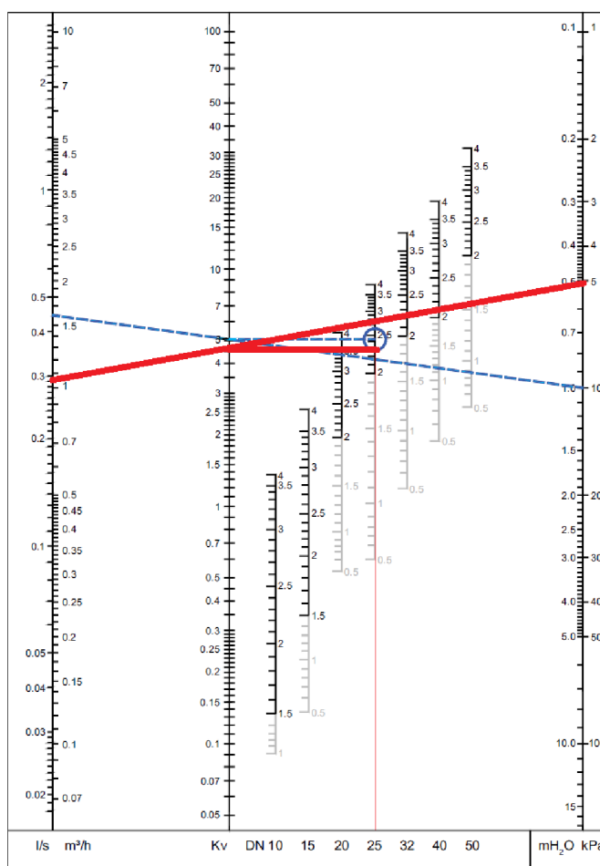
Obr. 40 Nastavení vyvažovacího ventilu na větvi č.1 [26]
