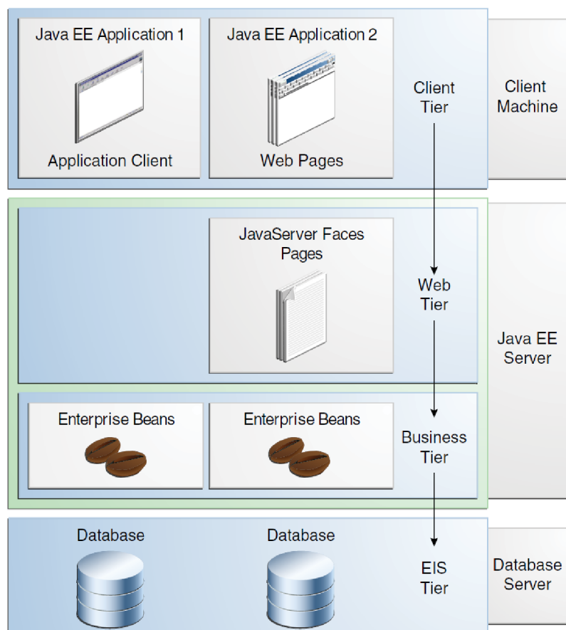
Obr. 2.3: Viacvrstvomá architektúra Java EE 8
