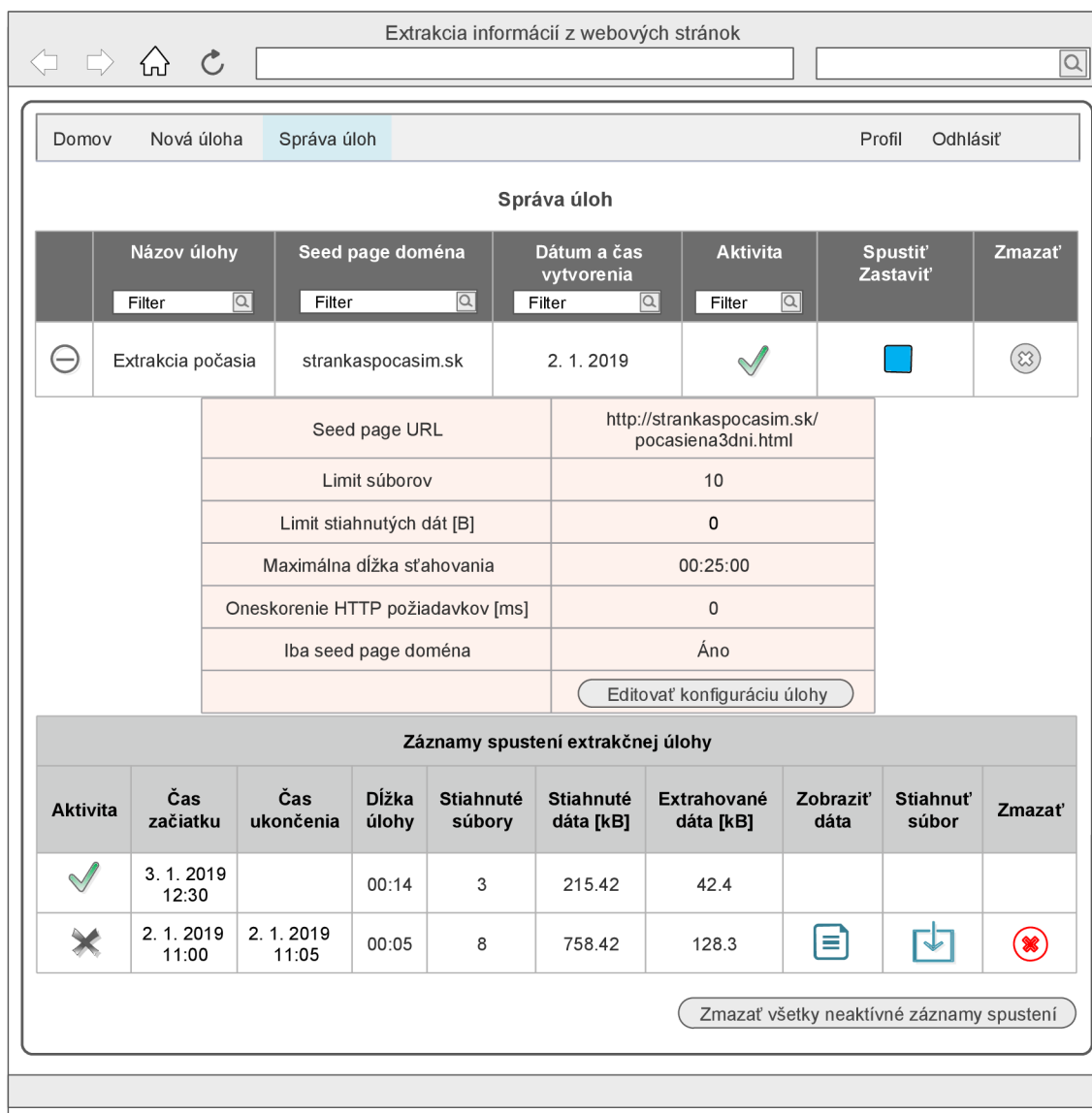
Obr. 4.11: Návrh GUI pre správu úloh – rozbalená úloha
