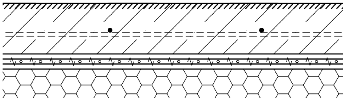
Obr. č. 43 DEK Hrubá podlaha [25]
