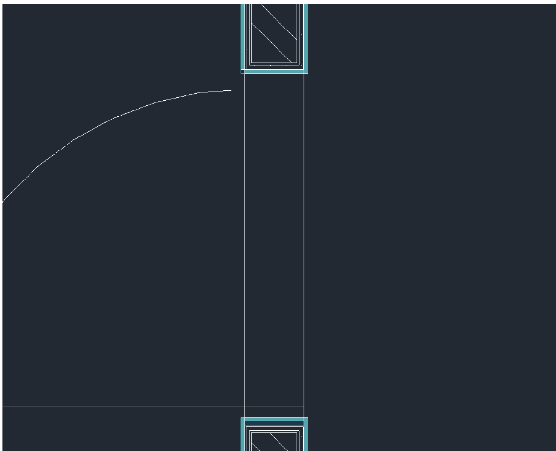
Obr. č. 32 Dilatační páska – Revit
