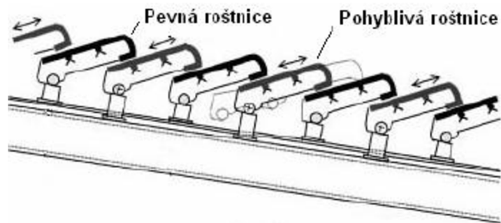
Obrázek 13: Posuvný rošt [8]
