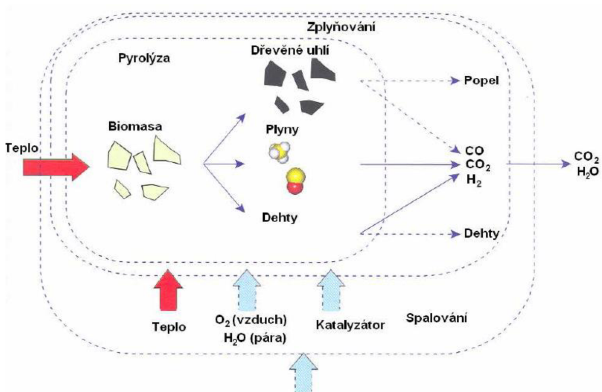
Obrázek 11: Schéma zplyňování [8]
