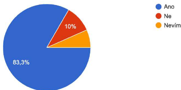
Obrázek 8. Graf: Otázka 6
