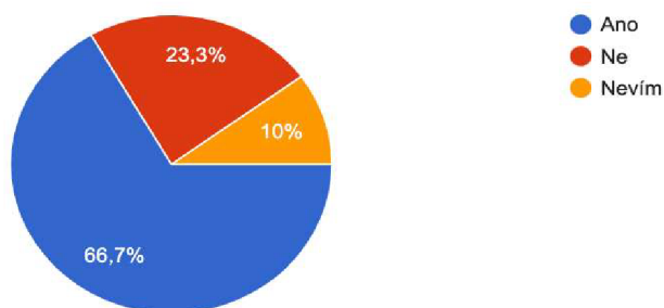
Obrázek 17. Graf: Otázka 14
