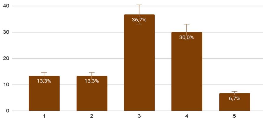
Obrázek 16. Graf: Otázka 13
