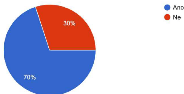
Obrázek 5. Graf: Otázka 3
