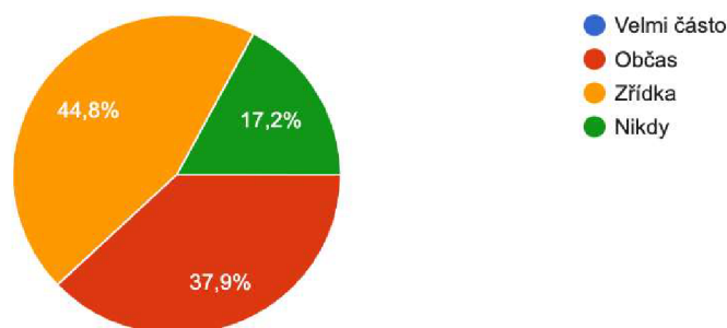
Obrázek 12. Graf: Otázka 9
