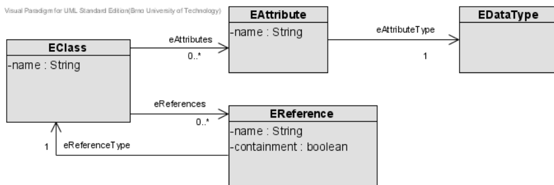
Obr. 3.2: Diagram tried zobrazuje zjednodušenú podmnožinu metamodelu Ecore [15].
