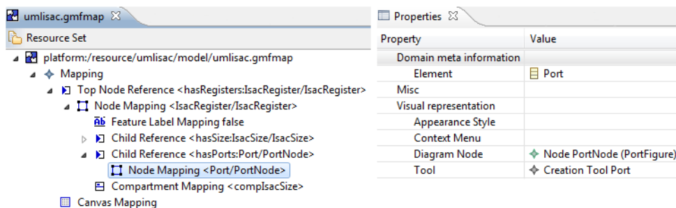
Obr. 6.4: Model mapovania.
