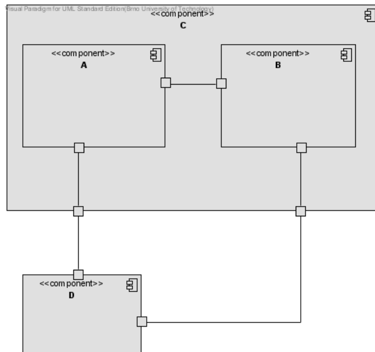
Obr. 2.1: Ukážka diagramu komponentov.
