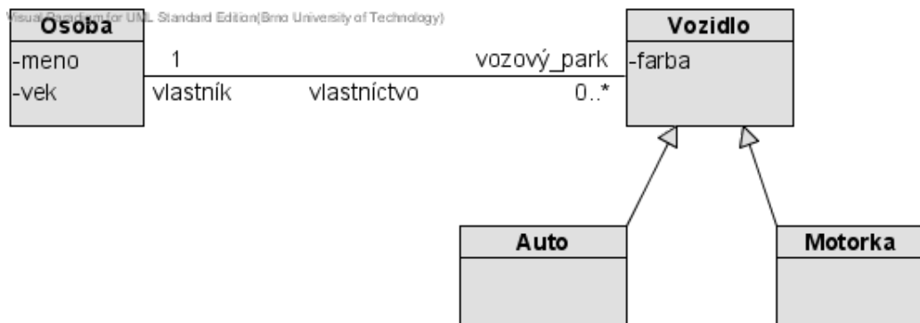
Obr. 2.6: Jednoduchý diagram tried na demoštrovanie použitia jazyka OCL. [6].
