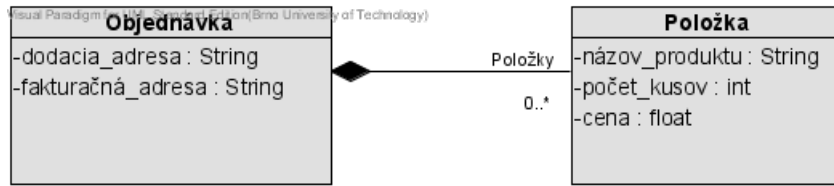
Obr. 3.1: UML diagram [15].
