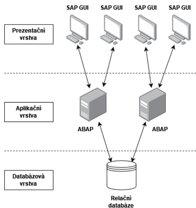
Obrázek 2.2: Architektura klient-server
