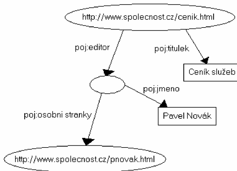
Obrázek 3.4 RDF graf
