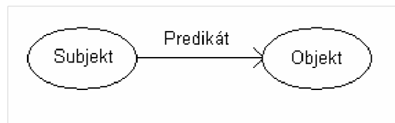
Obrázek 3.1 RDF trojice
