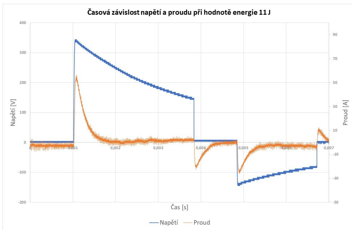
Graf 8 Časová závislost napětí a proudu při hodnotě napětí 11 J
