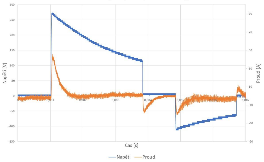
Časová závislost napětí a proudu při hodnotě energie 7 J
