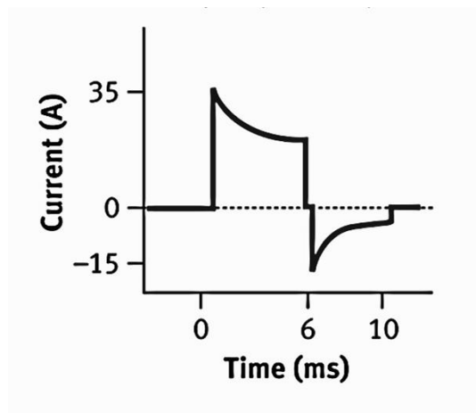
Obr. 8 Bifázický výboj – přímý (Young and Harrison, 2021)
