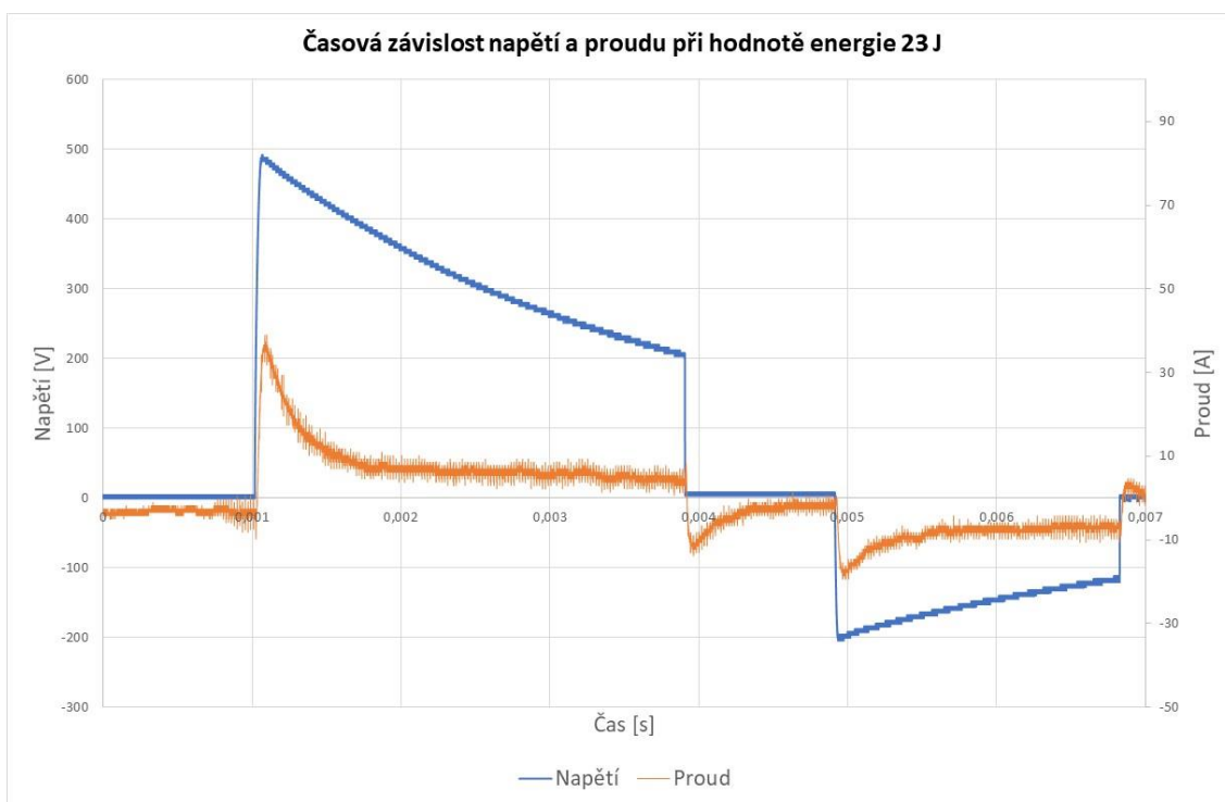
Graf 9 Časová závislost napětí a proudu při hodnotě energie 23 J
