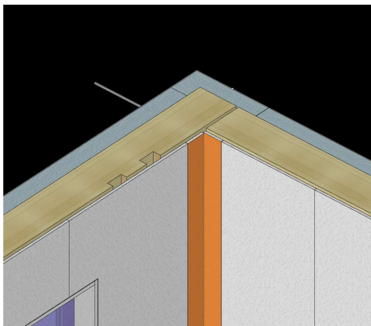
Obrázek 16 Napojení obvodových panelů
