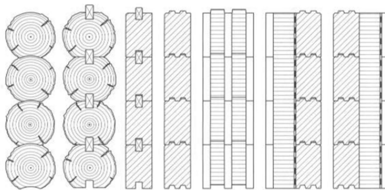
Obrázek 3 Druhy vodorovných prvků srubu
