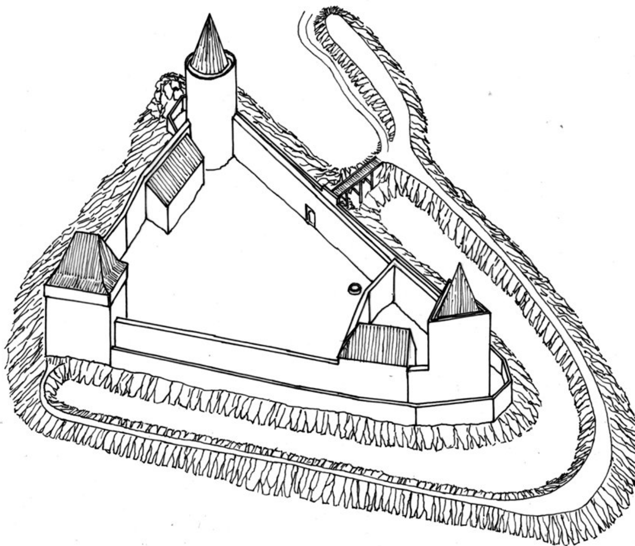
Obr. 12: Hmotová rekonstrukce hradu Lichnice. Pravděpodobný stav k roku 1300. Autor Miroslav Plaček.
