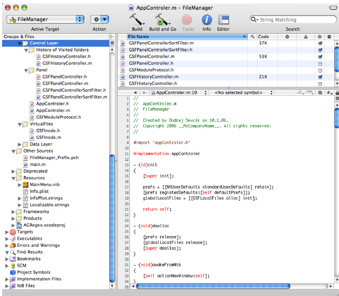
Obrázek 3.3: Project Builder
