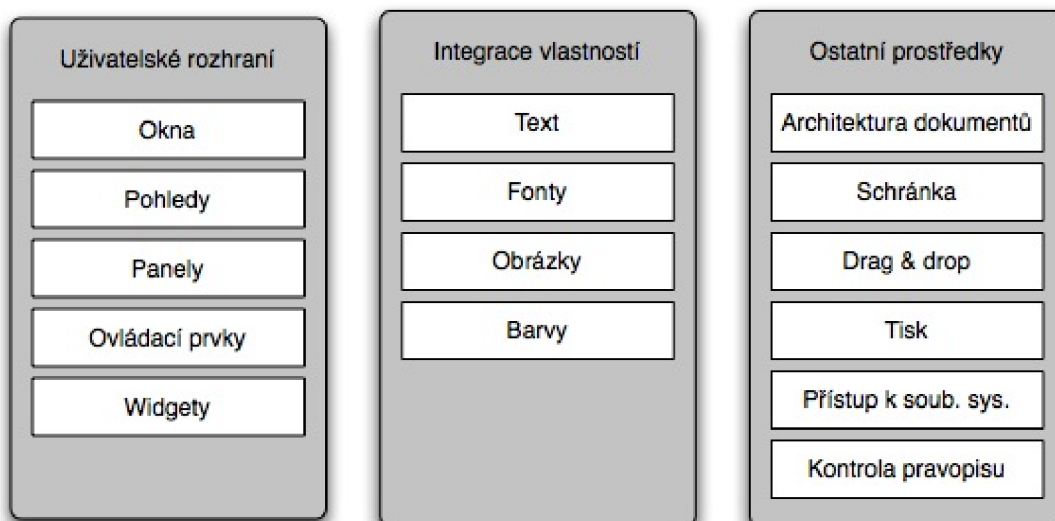
Obrázek 3.2: Application Kit
