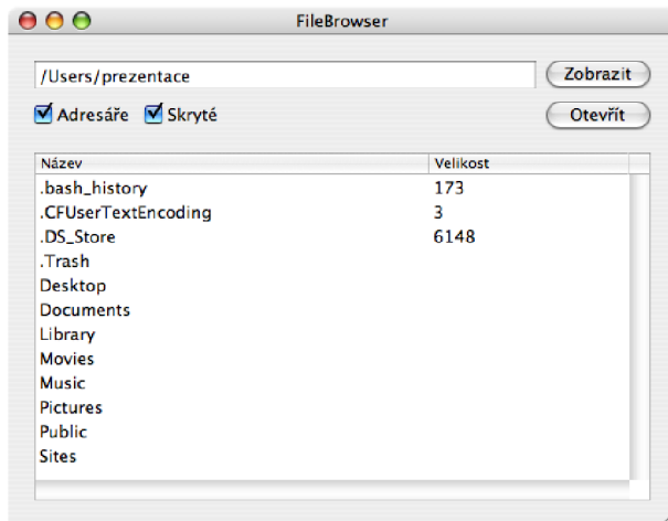
Obrázek 3.7: Aplikace FileBrowser
