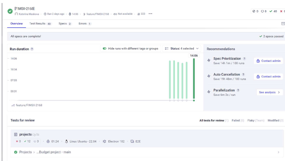
Obrázek 12 Ukázka testovacího běhu v Cypress Dashboardu
