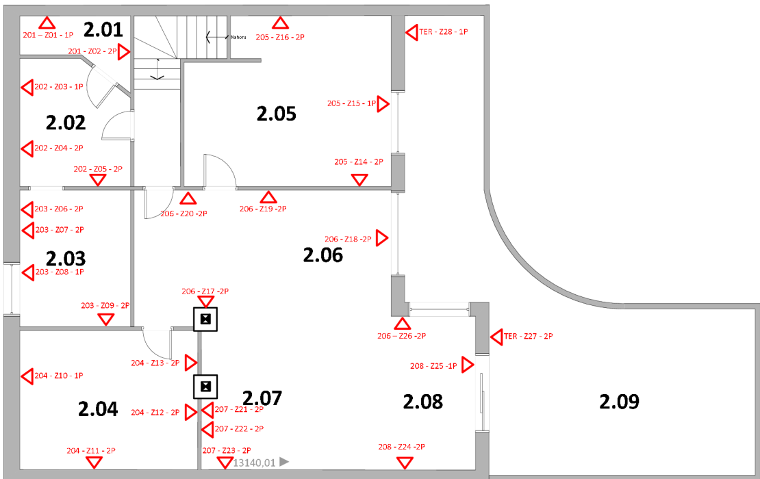
Nákres 3: Koncové body - Prvé poschodie
