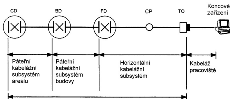
Obrázok 8: Schematické zobrazenie štruktúry univerzálnej kabeláže
