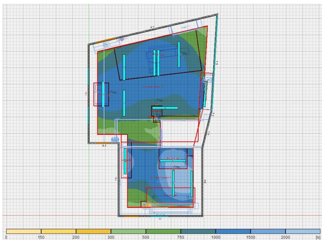
Obrázek 3-3 Návrh 2 - intenzita osvětlení
