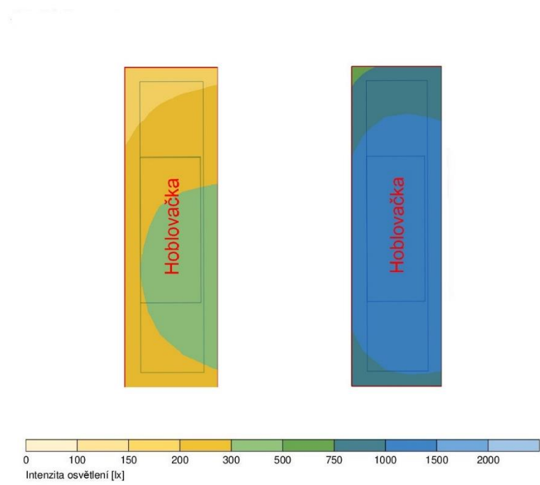
Obrázek 4-8 Porovnání hoblovačka
