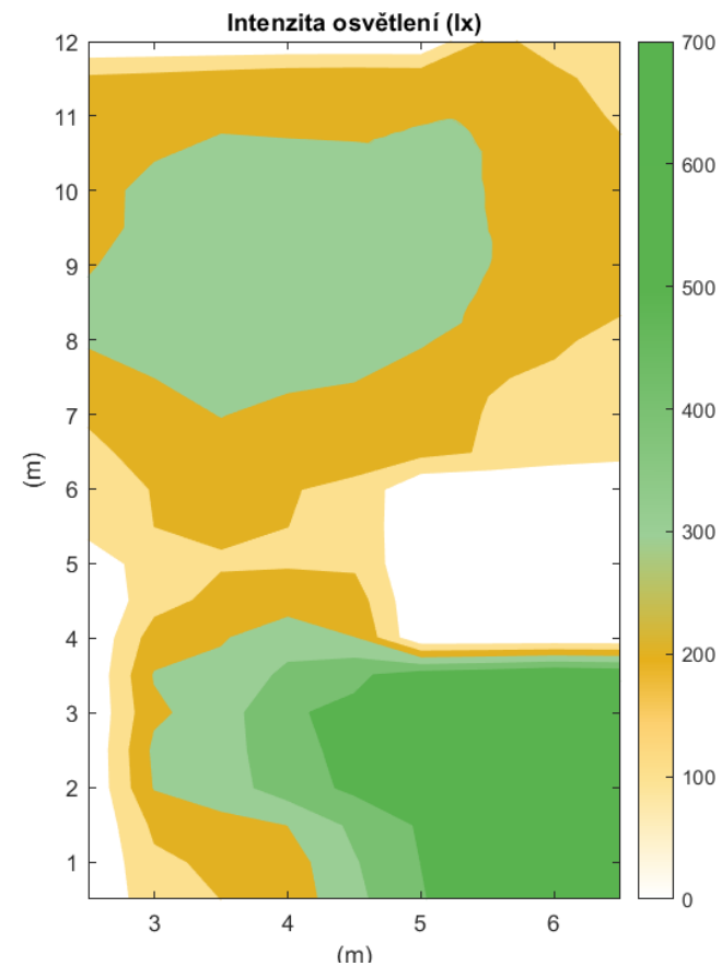
Obrázek 2-6 Naměřené hodnoty
