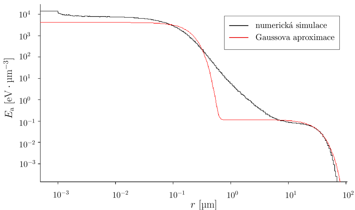
Obr. 2.4: Numerický model PSF funkce a její Gaussova aproximace u dna rezistu PMMA o tloušťce w = 2,5 \mu\text{m} na Si podložce a pro počáteční energii elektronů E_0 = 100 \text{ keV} . Gaussovou aproximací získány hodnoty parametrů: \alpha = 0,186 \mu\text{m} , \beta = 30,46 \mu\text{m} a \eta = 0,74 .
