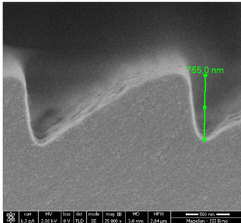
Obr. 4.18: Měření hloubky mřížky na SEM. Transmisní mřížka naladěná na 1. řád. \Lambda = 2 \mu\text{m} , N = 10 .
