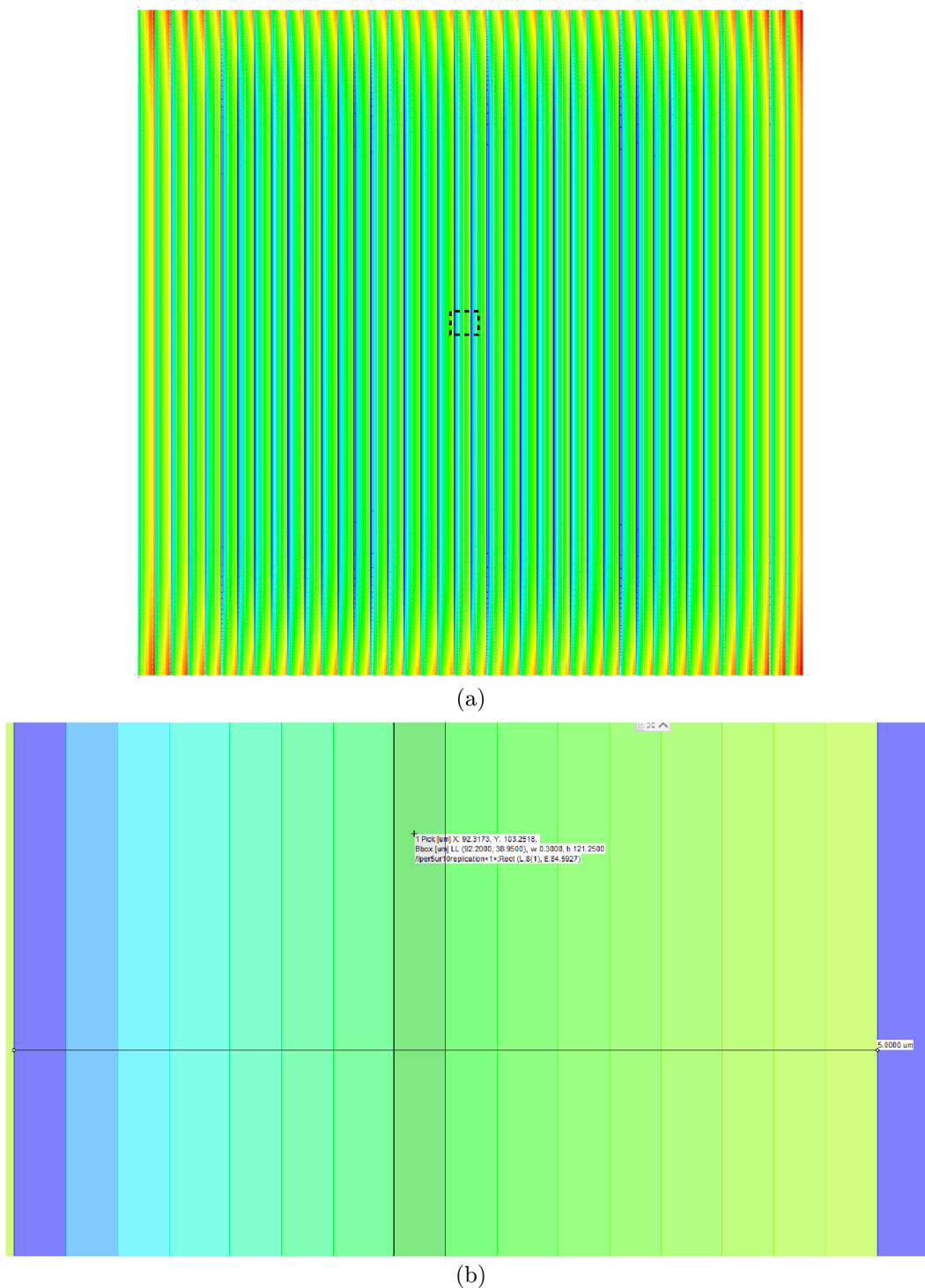
Obr. 4.16: Výsledek výpočtu modulu 3D-PEC pro transmisní blejzovanou mřížku naladěnou na první řád s parametry: \Lambda = 5 \mu\text{m} a N = 16 . (a) Celé pole (rozměr 200 \times 200 \mu\text{m} ). (b) Detail o velikosti jedné periody s ukázkou odečtení expoziční dávky pro úroveň č. 8.
