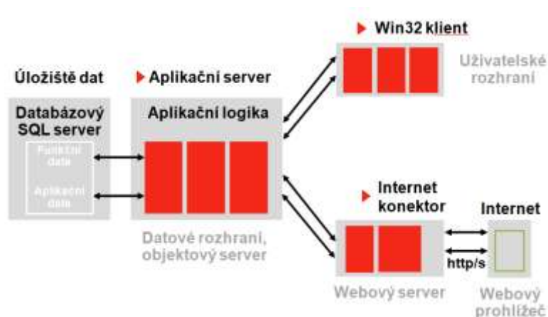
Obr. 17 - Architektura QI 106
