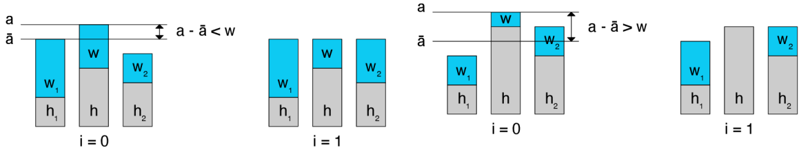
Obrázek 3.5: Prípád 2: aktuálna baunka obsahuje menej vody, než je potrebné pre vyrovnanie celkovej výšky susedných buniek a distribuje celý svoj objem vody. Inšpirované z [7].
