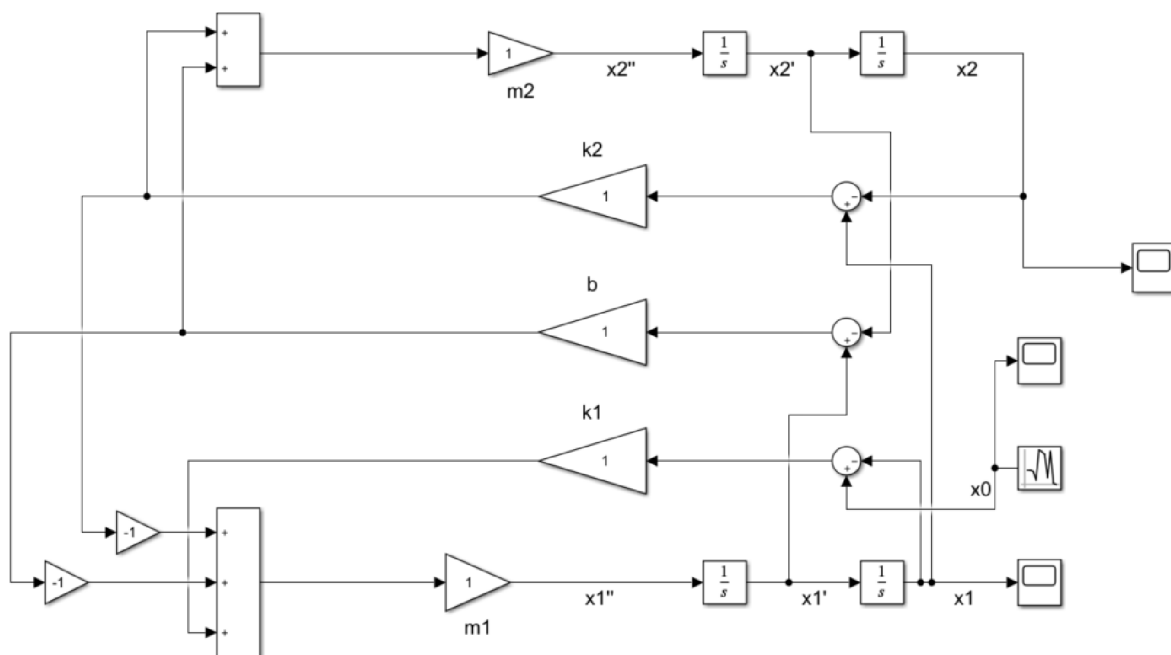
Obr. 35 Štvrtinový model vozidla v softvéri MATLAB/Simulink
