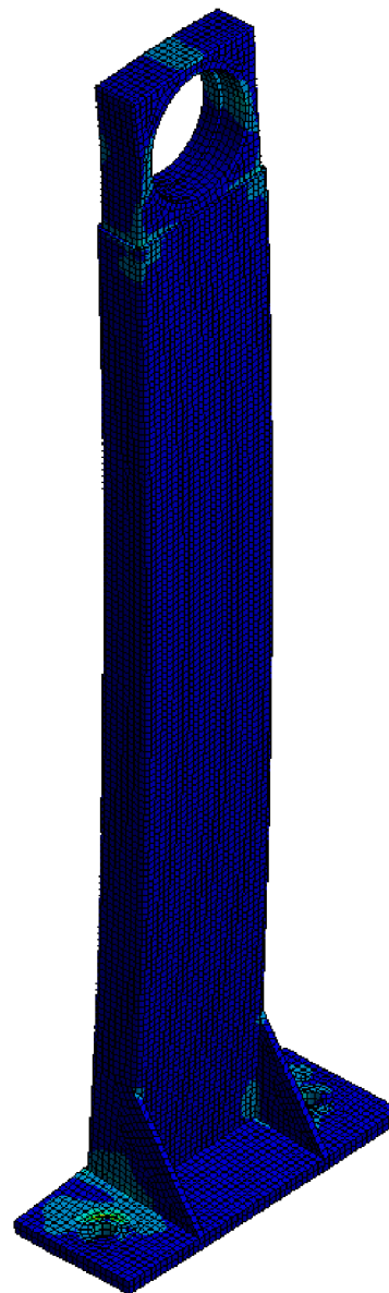
Obr. 28 Rozloženie výsledného napätia
