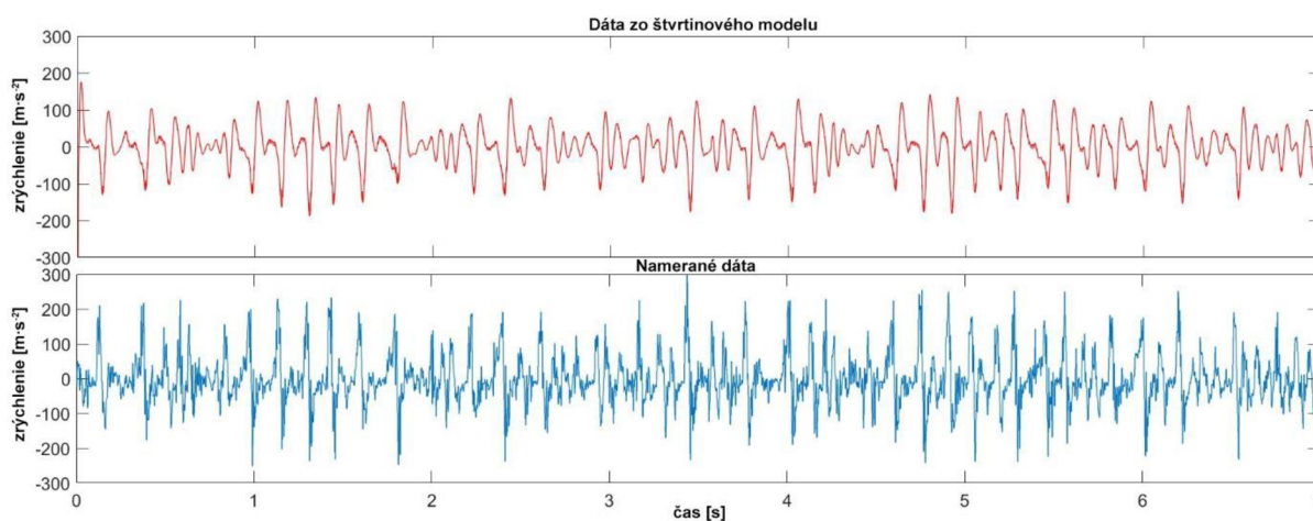
Obr. 43 Porovnanie zrýchlení neodpružených hmôt zo štvrtinového modelu a reálne nameraných
