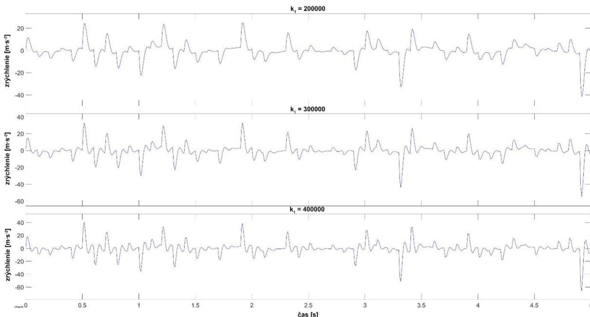
Obr. 38 Zrýchlenia odpružených hmôt pre rôzne tuhosti pneumatiky
