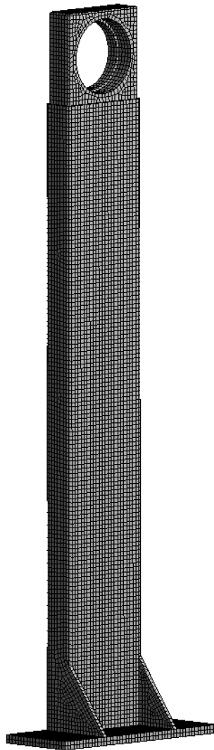
Obr. 24 Sieť použitá pre výpočet
