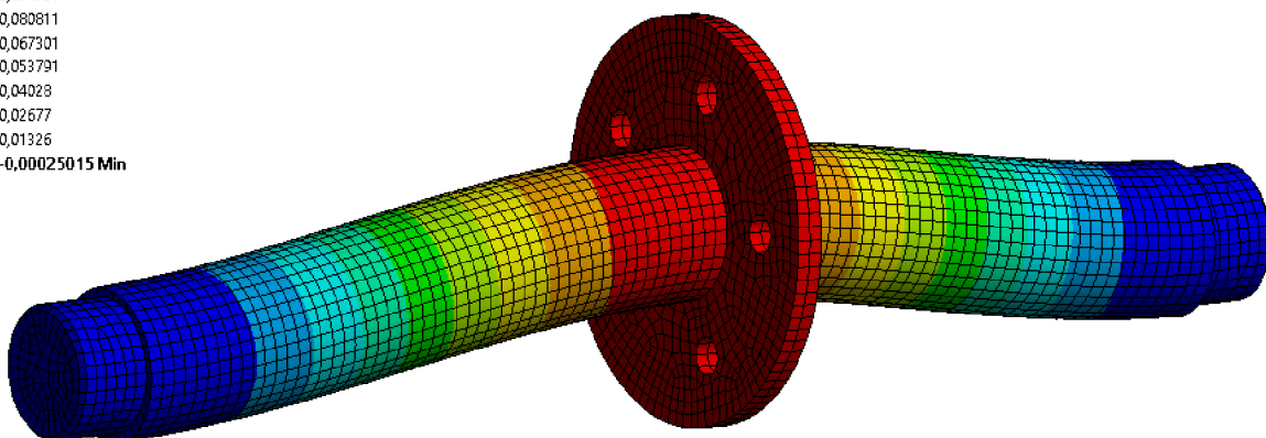
Obr. 31 Deformácia v osi zaťaženia
