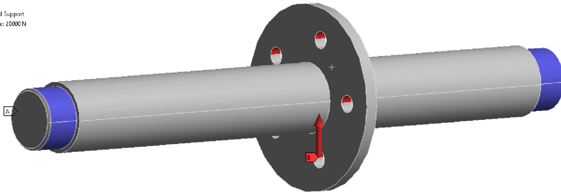
Obr. 30 Miesta uchytenia a pôsobiská zaťažovacej sily
