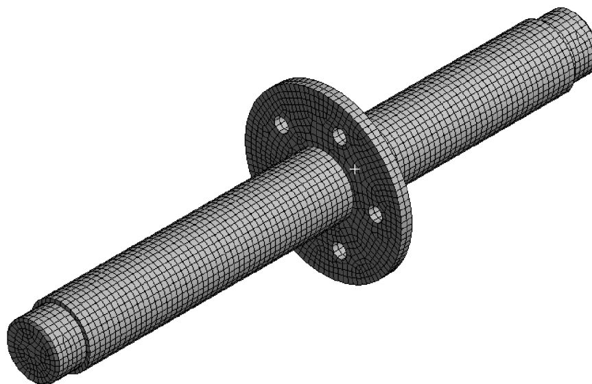
Obr. 29 Sieť použitá pre výpočet
