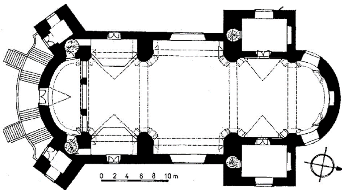
Obr. 2: Púdorys kostela
