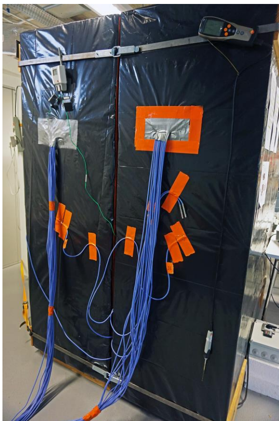
Příloha 7: Teplá skřín z boku po osazení testovaného panelu a uzavření obou komor ocelovými pásky; vpravo teplá komora, vlevo chladná komota
