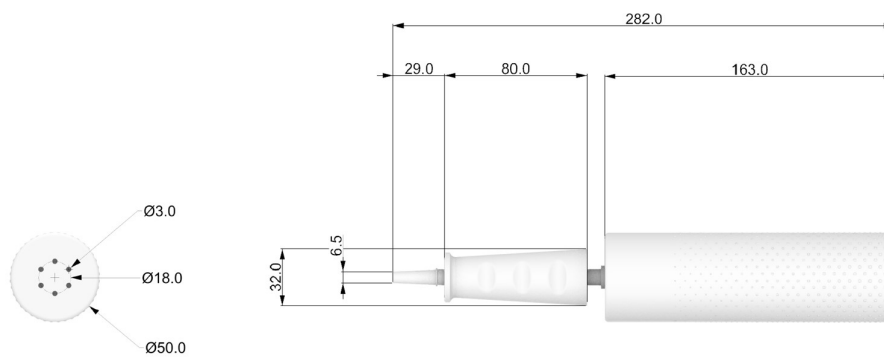
Obr. 6-4 Rozměry pumpičky (M 1:4)
