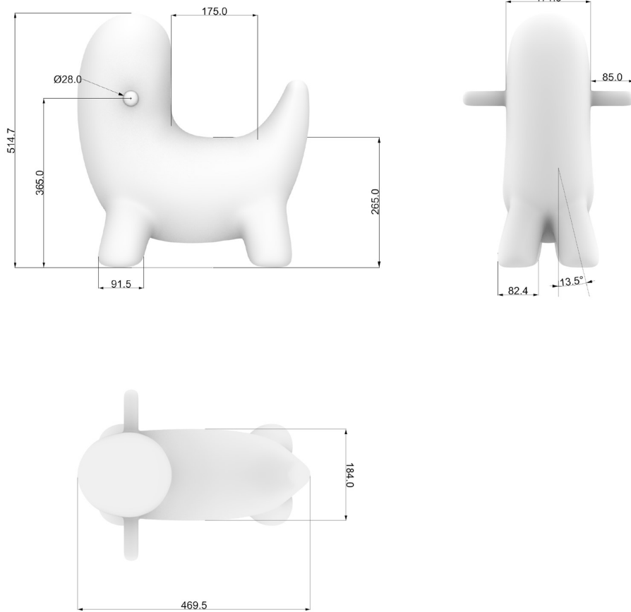
Obr. 6-1 Rozměry prvního skákadla (M 1:10)
