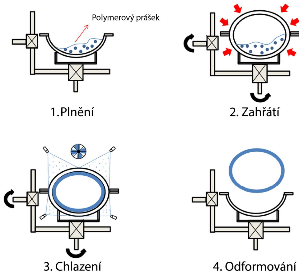
Obr. 2-14 Schéma rotačního tváření plastů [18]
