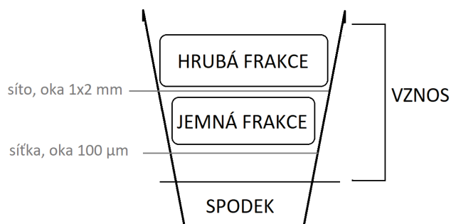
obr. 12 - Diagram zobrazující frakce, jako nadsítné a podsítné daných sít a vztahu vzosu a spodku
