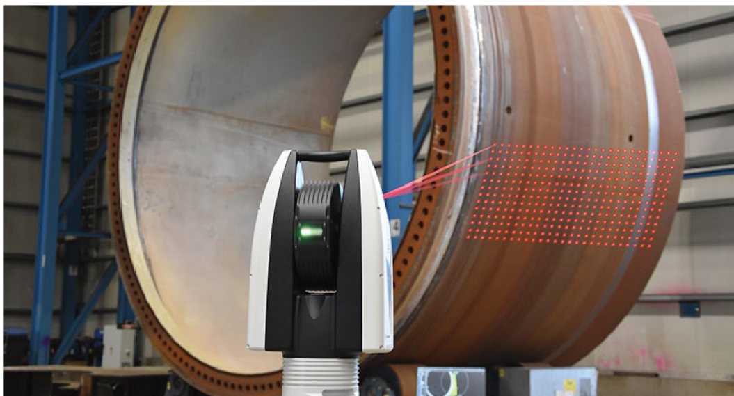
Obr. 9 Leica Absolute Tracker ATS600 umožňuje vykonávať laserové merania bez laserových terčov, priamo z laserového systému snímacieho zariadenia. [5]
