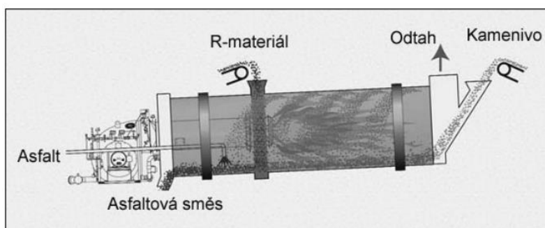
Obrázok č. 16: Pridávanie R-materiálu proti prúdu horúceho vzduchu [10]
