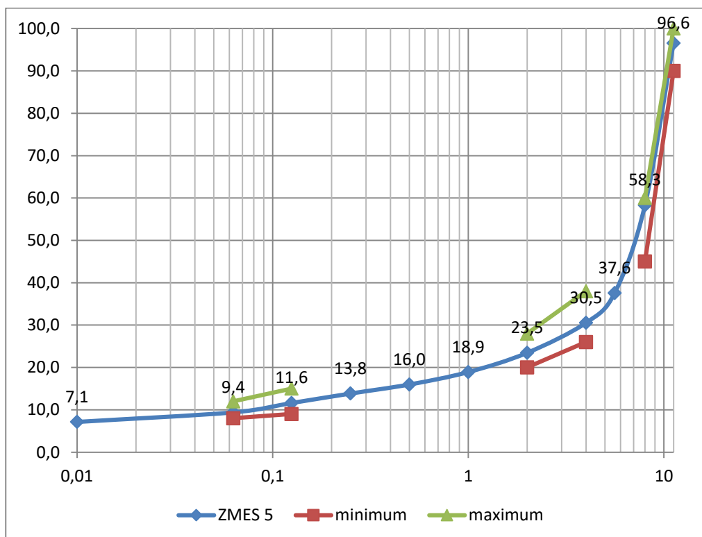
Graf č. 2: Zrornosť zmesi 5 s limitnými hodnotami pre SMA 11 S podľa EN 13108-5
