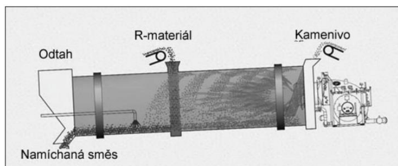
Obrázok č. 15: Pridávanie R-materiálu súbežne s prúdom horúceho vzduchu [10]
