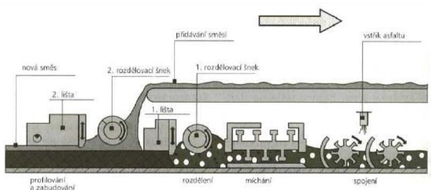
Obrázok č. 4: Princíp technológie Remix Plus [7]
