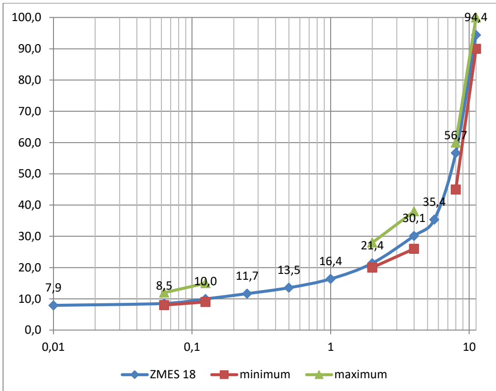
Graf č. 5: Zrinitosť zmesi 18 s limitnými hodnotami pre SMA 11 S podľa EN 13108-5
