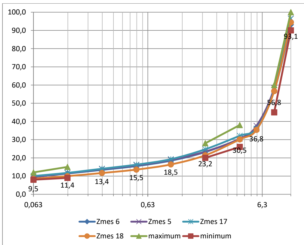
Graf č. 6: Zrinitosť zmesí s limitnými hodnotami pre SMA 11 S podľa EN 13108-5
