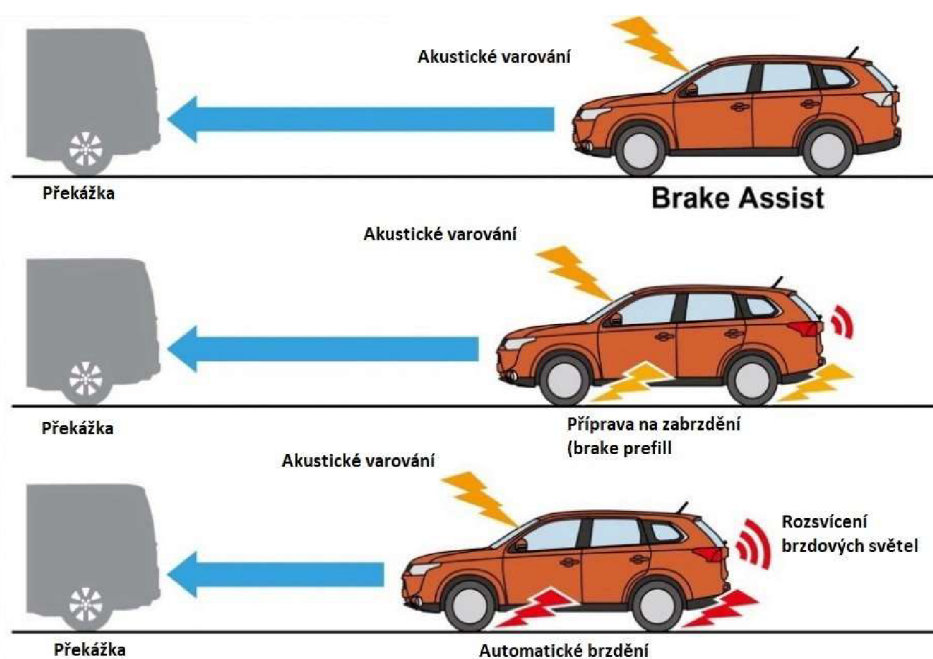
Obrázek 9 - Ukázka funkce systému FCW (42)
