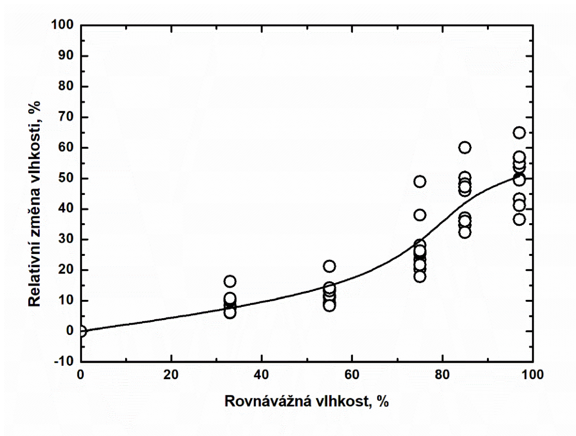
Obr. 22 Desorpční izoterma analyzovaného druhu biocharu.
