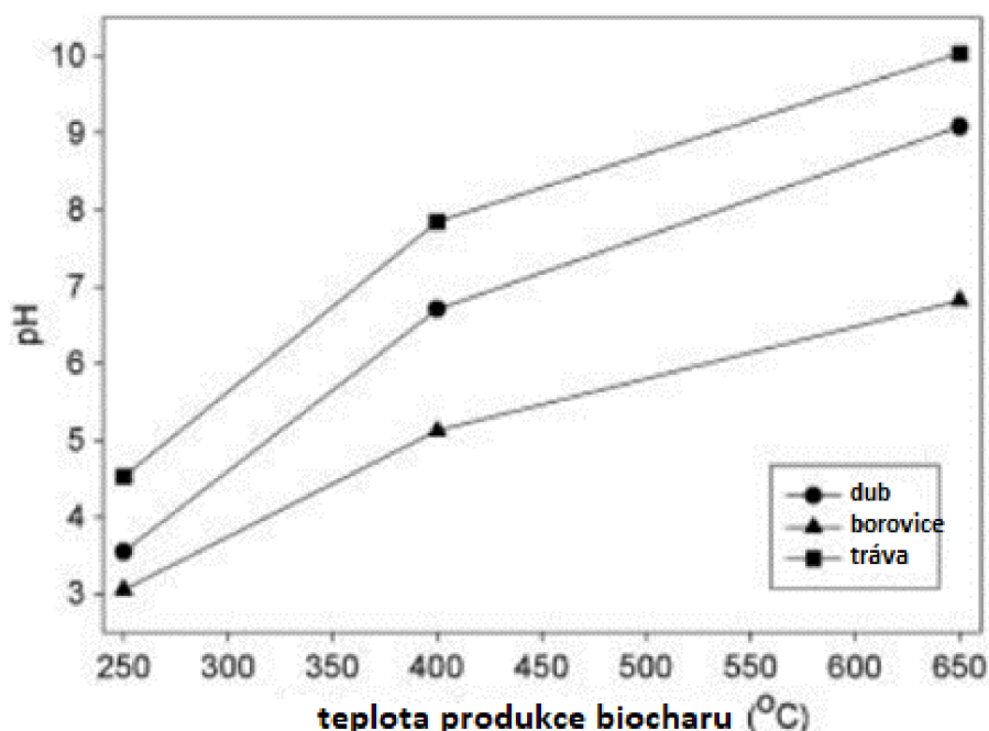
Obr. 15 Závislost hodnot pH biocharu na pyrolýzní teplotě. [50]
