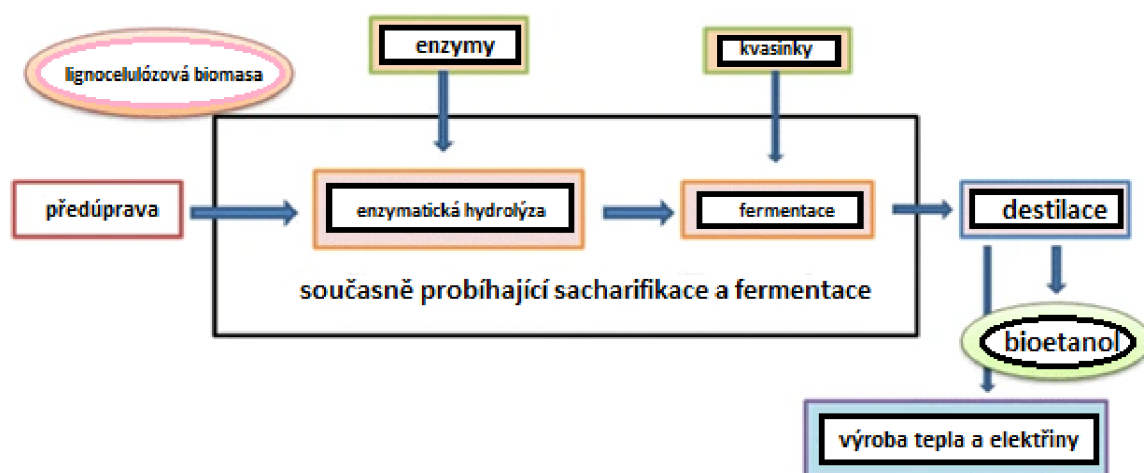
Obr. 11 Biologická přeměna lignocelulózové biomasy na bioethanol. [36]
