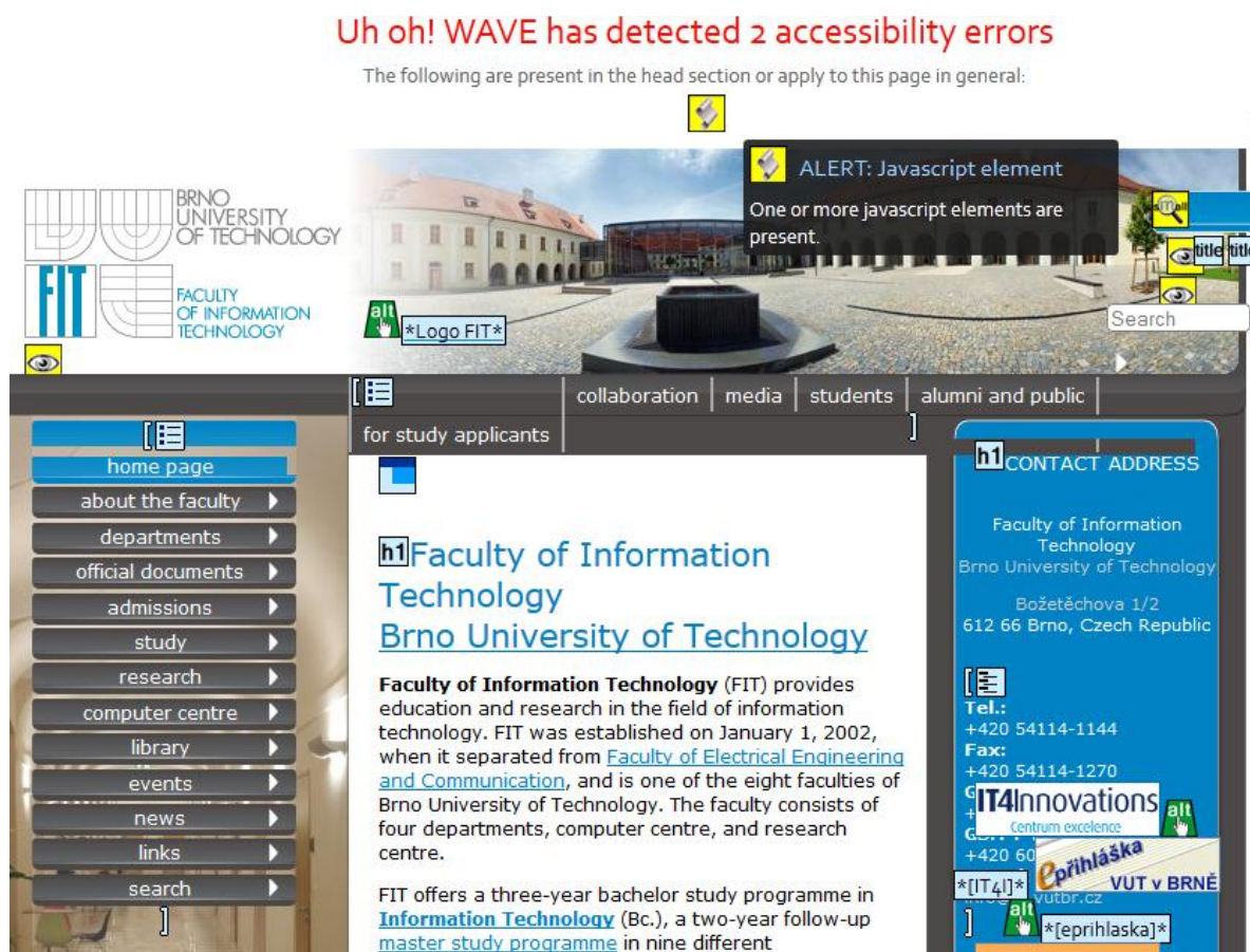
Obrázok 5.2: Grafický výstup validácie webovej stránky www.fit.vutbr.cz
