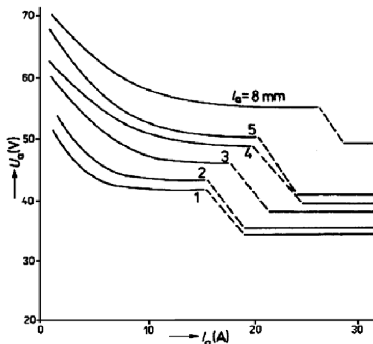
Obr. 6 Charakteristiky elektrických oblouků změřené Ayrtonovou
