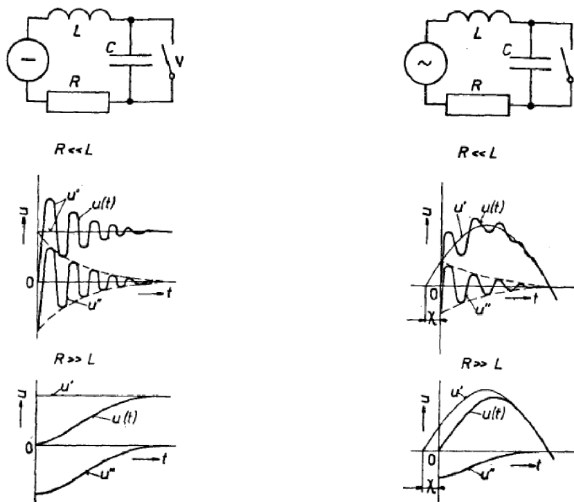
Obr. 3 Vypínání v stejnosměrném a ve střídavém obvodě
