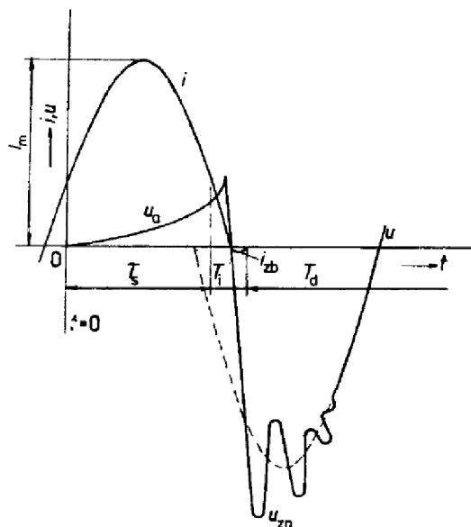
Obr. 11 Zhášení střídavého oblouku
