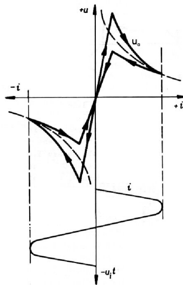
Obr. 9 Dynamická voltampérová charakteristika
