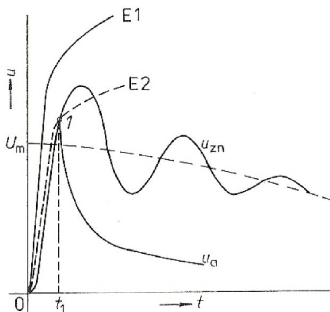
Obr. 12 Podmínky úspěšného uhasnutí oblouku
