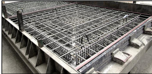
Obr. 7 Kompozitní výztuž zákrytové desky v bednění před betonáží
