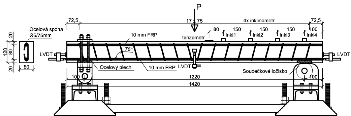
Obr. 6 Schéma nosíkové únavové zkoušky
